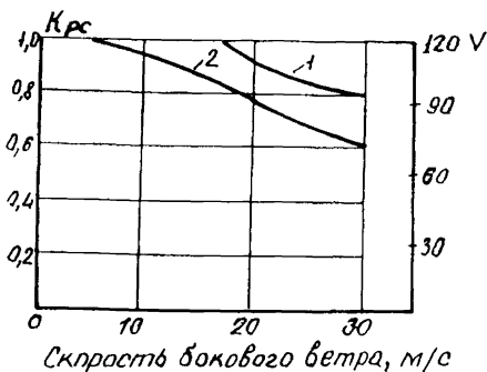
Рис. 10. Зависимость коэффициента снижения расчетной и допустимой скорости движения одиночного автомобиля от скорости бокового ветра:
