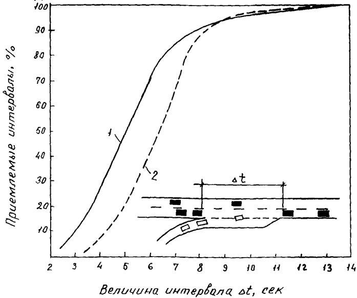
Рис. 2. Распределение величин приемлемых интервалов при въезде автомобилей на магистраль: 1 - соходу; 2 - после остановки
