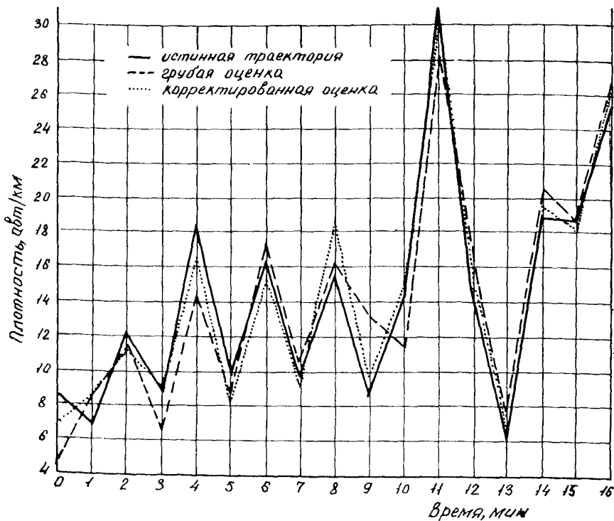
Рис.12. Результаты оценивания плотности транспортного потока на одной из полос шестиполосного участка магистрали ниях элементов, следующих ковариационных матриц:
