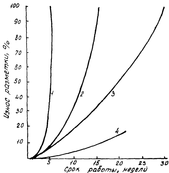
Рис. I. Износостойчивость разметки из различных материалов: 1 - краски на основе алкидных смол; 2 - краски на основе алкидных смол и хлоркаучука; 3 - краски на основе хлоркаучука; 4 - термопластики
