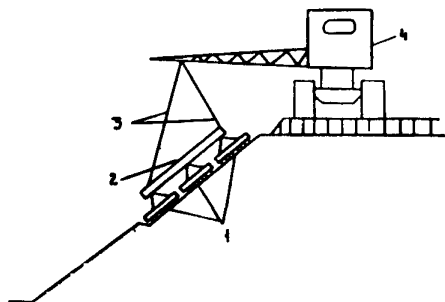
Рис.8. Схема установки комплекта борон: 1-бороны; 2-траверса; 3-тросы; 4-трактор
