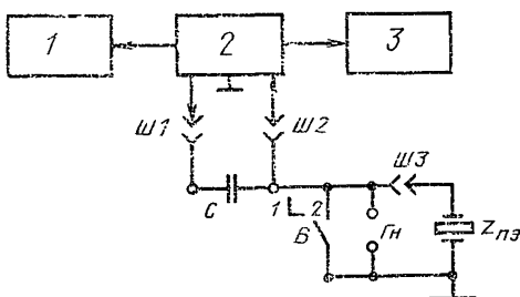
1 — частотомер; 2 — измеритель АЧХ; 3 — графопостроитель
