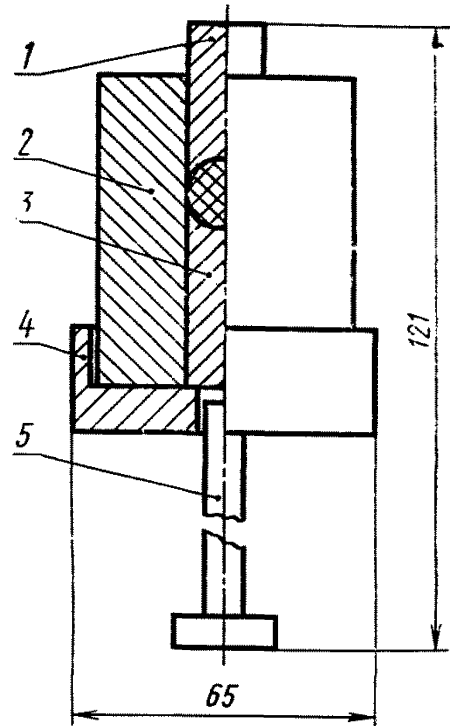
1 — пуансон верхний; 2 — обойма; 3 — пуансон нижний; 4 — основание; 5 — выталкиватель
