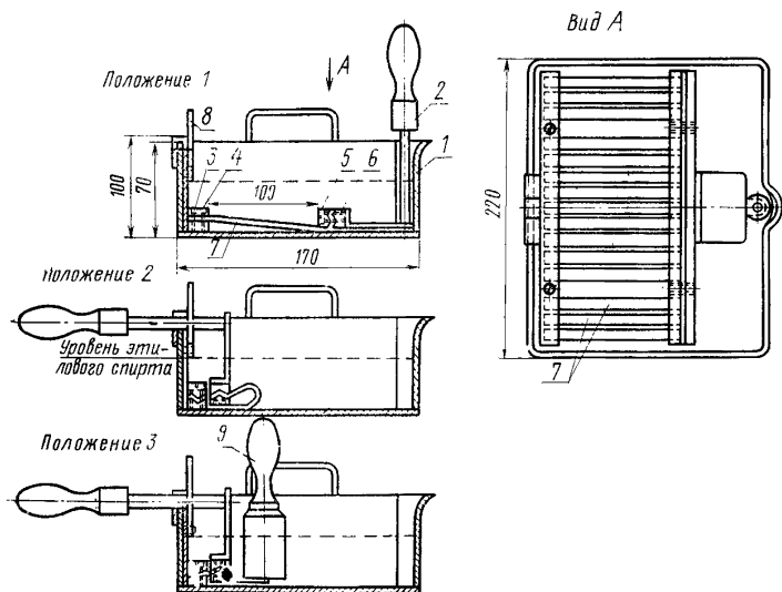
1—ванна; 2—ручка; 3—зажим № 1; 4, 6—бруски; 5—зажим № 2; 7—образцы; 8—защелка; 9—пестик.
