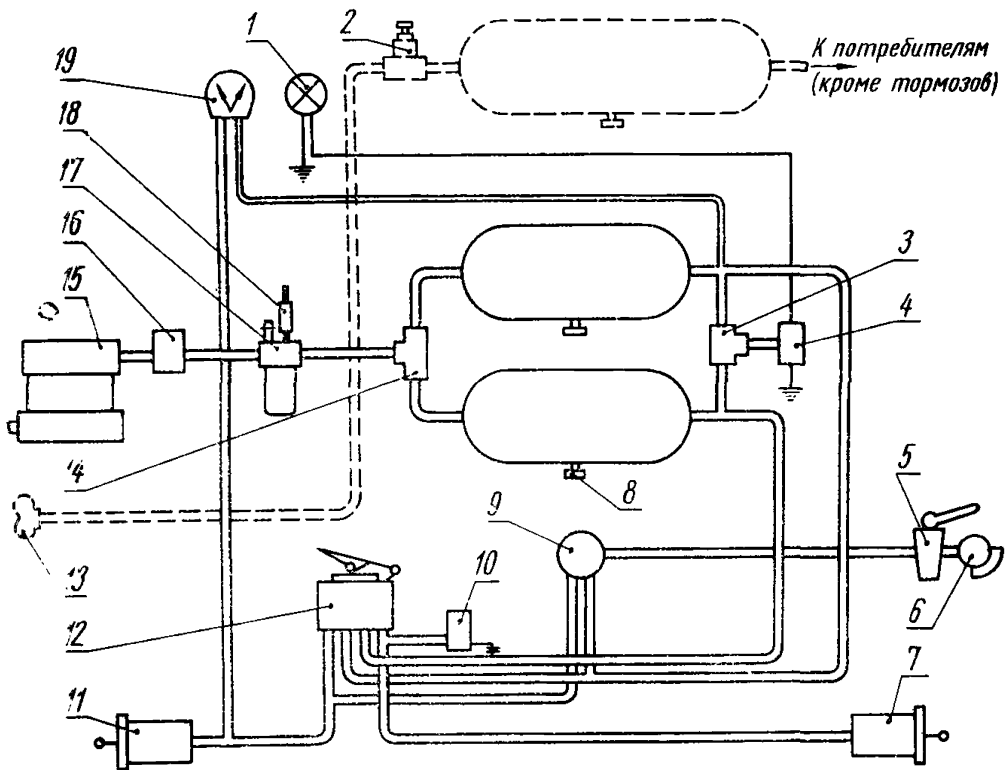
1— сигнальная лампочка; 2—перепускной клапан; 3 — двойной клапан-ограничитель; 4—выключатель сигнальной лампы; 5—разобщительный кран; 6 — соединительная головка типа А; 7—рабочие органы тормозов колес; 8—спускной кран; 9 — тормозной кран прицепа; 10 — включатель стоп-сигнала; 11 — рабочие органы тормозов передних колес; 12 — тормозной кран автомобиля; 13 — буксирный клапан; 14 — двойной защитный клапан; 15 — компрессор; 16 — регулятор давления; 17 — влагомаслоотделитель и кран отбора воздуха; 18 — предохранительный клапан; 19 — двухстрелочный манометр.
