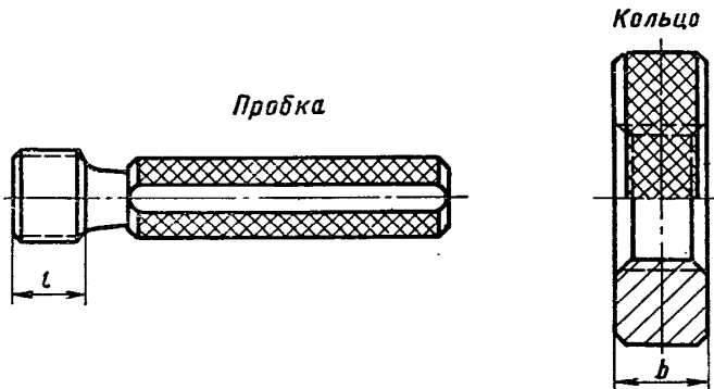
а) Для метрических резьб по ГОСТ 9150—59
