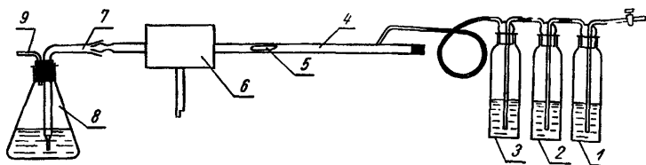
1, 2, 3 — склянки Дрекслея; 4 — кварцевая трубка со шлифом; 5 — фарфоровая лодочка; 6 — электрическая печь; 7 — кварцевое колено; 8 — приемник; 9 — отводная трубка к насосу.
