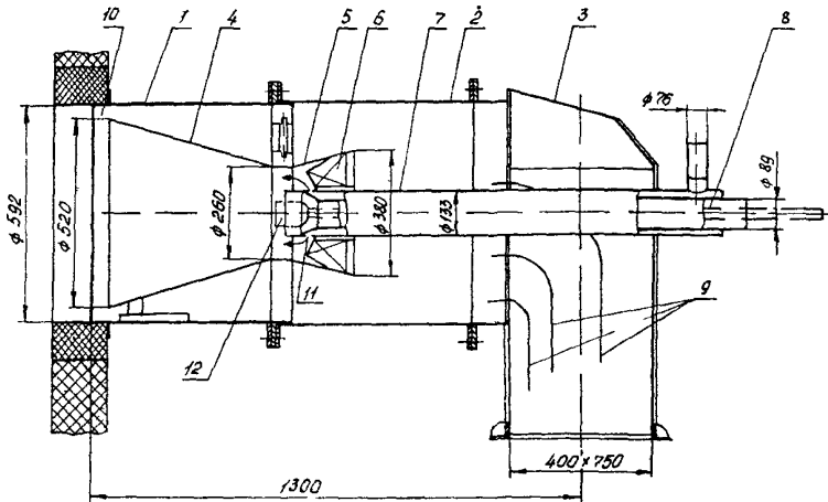
Рис.2. Надподовая горелка для плавки шлака (II вариант)
