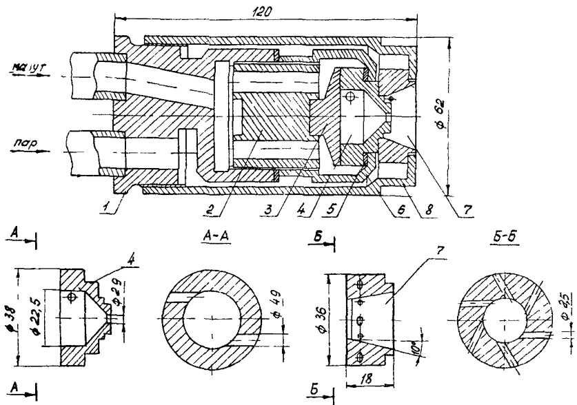
Рис.3. Паромеханическая форсунка
