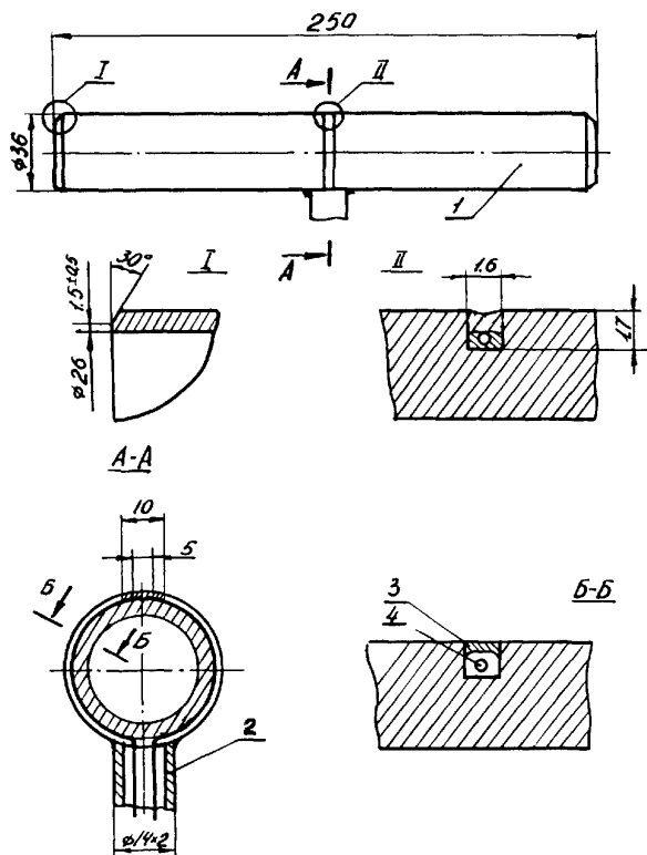
Рис.1. Температурная вставка с поперечной проточкой: 1 - вставка; 2 - защитная труба; 3 - профильная фольга; 4 - термопреобразователь
