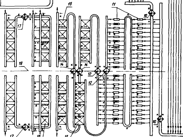
Рис. П.1. Схема экспериментального контроля пароперегревателей головного котла ТМЕ-206:
