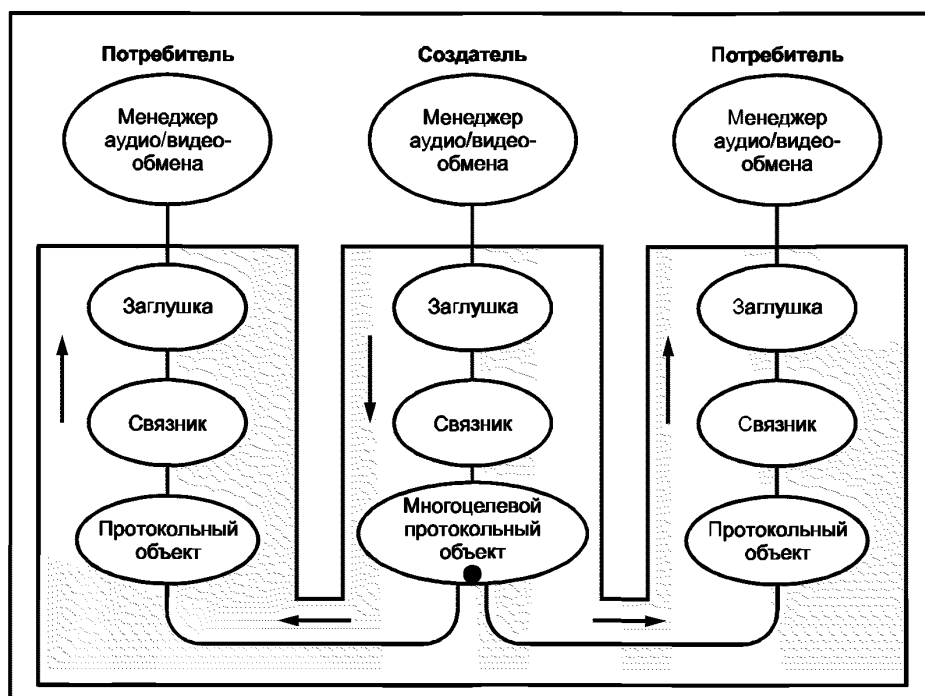
Рисунок 29 — Многоконечный канал для потока 2
