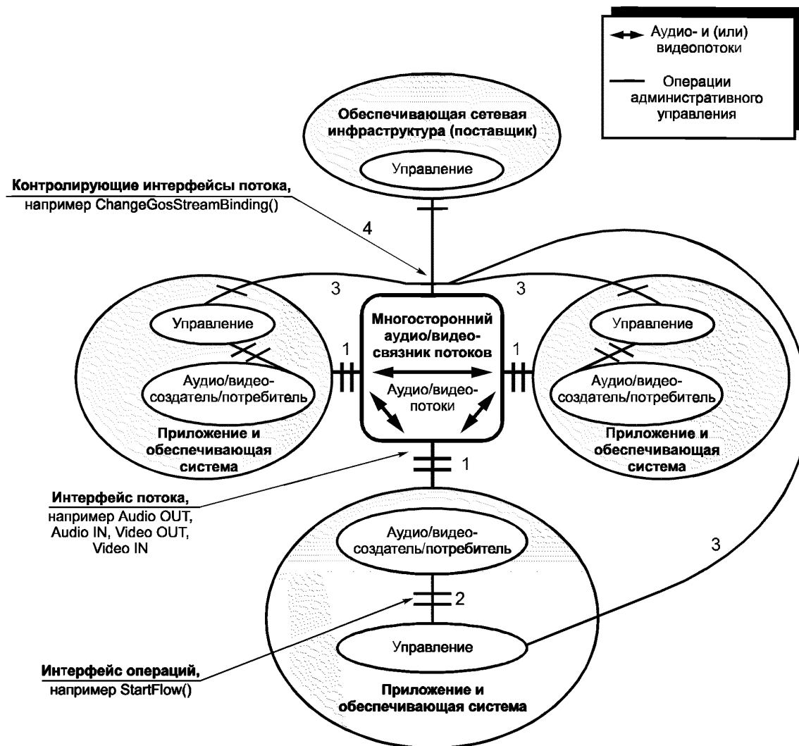
Рисунок 30 — Многостороннее связывание аудио/видеопотоков
