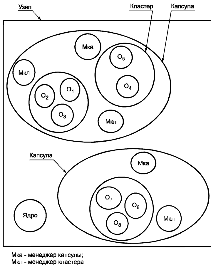
Рисунок 3 — Капсулы, кластеры и узлы
