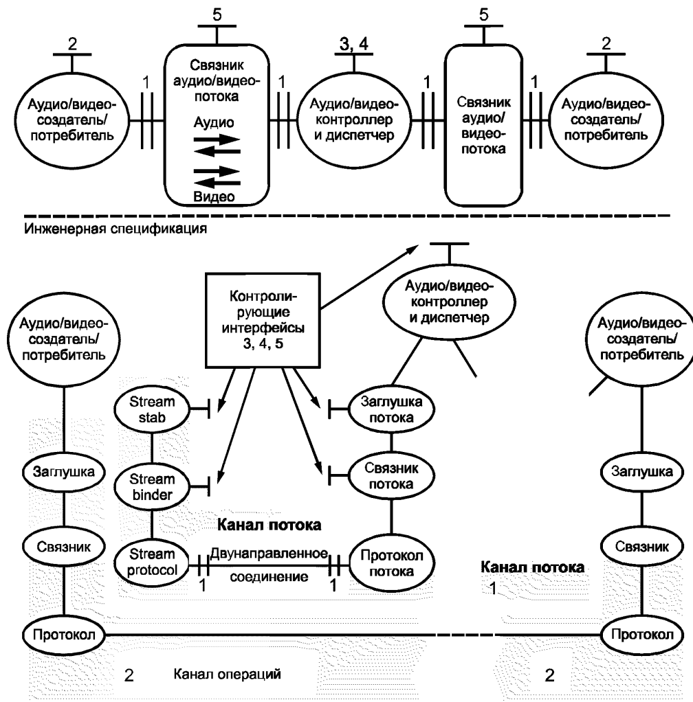
Рисунок 35 — Отображение вычислительной спецификации в инженерную
