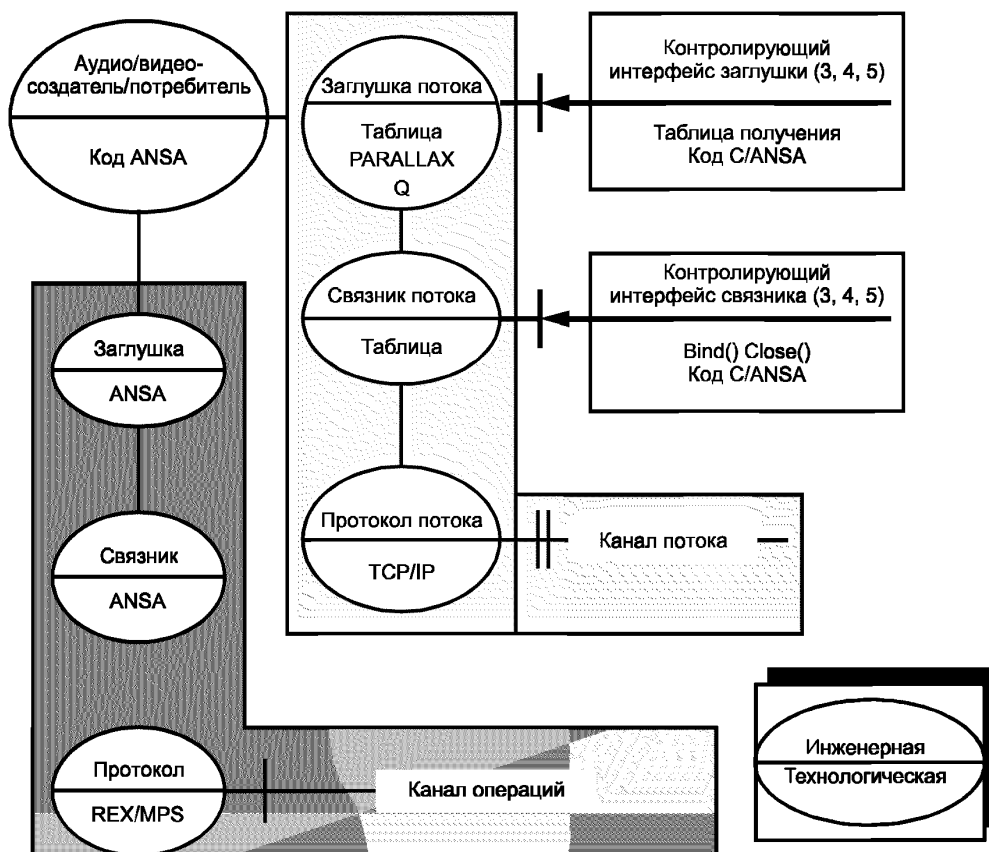
Рисунок 36 — Отображение инженерной спецификации в технологическую
