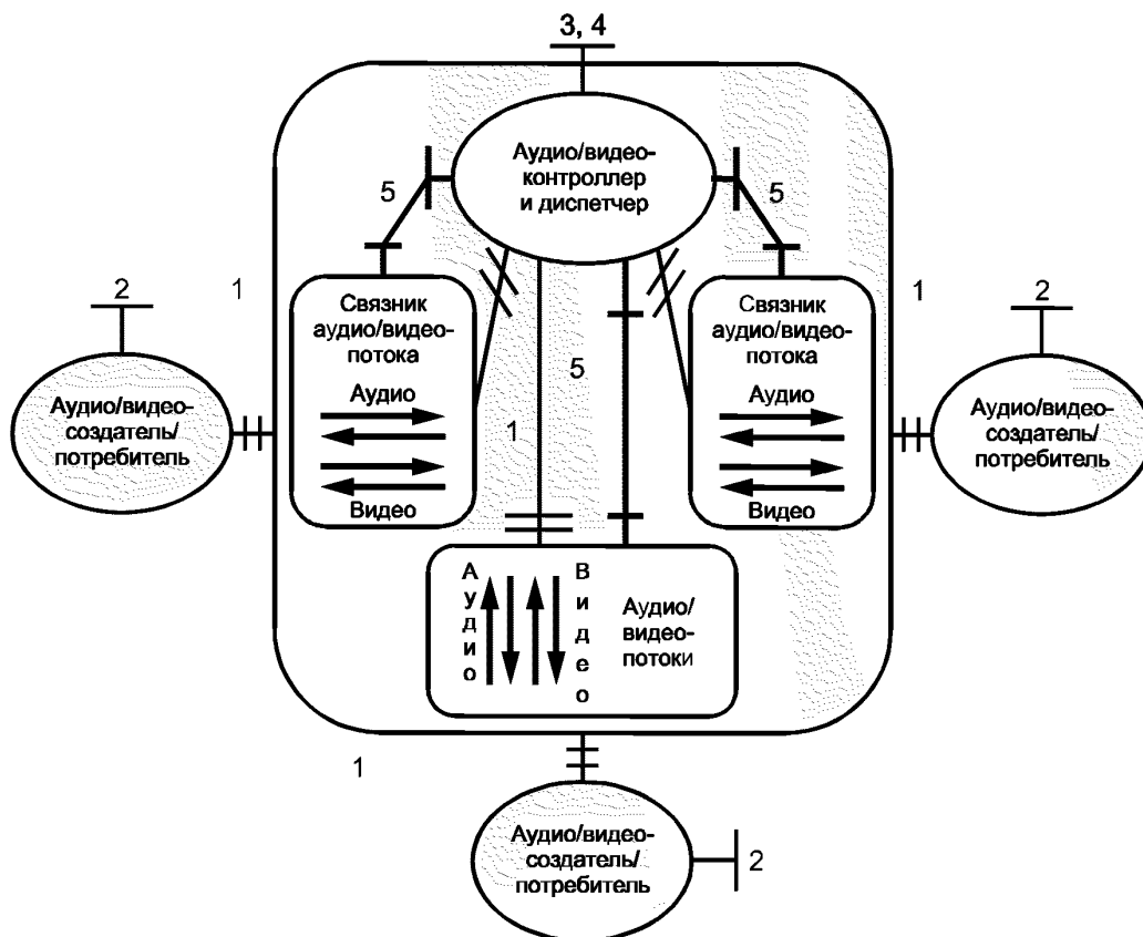
Рисунок 34 — Объекты, участвующие в многостороннем аудио/видеообмене
