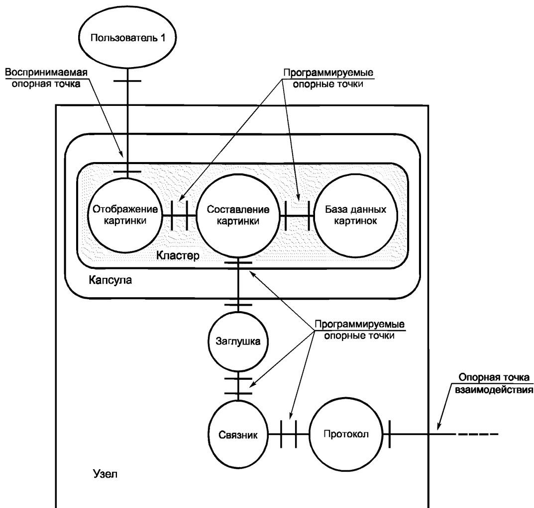
Рисунок 19 — Инженерная точка зрения (часть)
