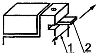
1 — направления усилия; 2 — рычаг привода механизма регулирования высоты пламени
