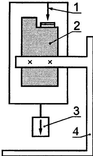
1 — направление усилия для искрообразования; 2 — корпус зажигалки; 3 — груз; 4 — штатив
