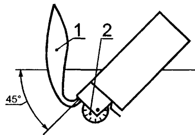
1 — пламя; 2 — искробразующее колесико
