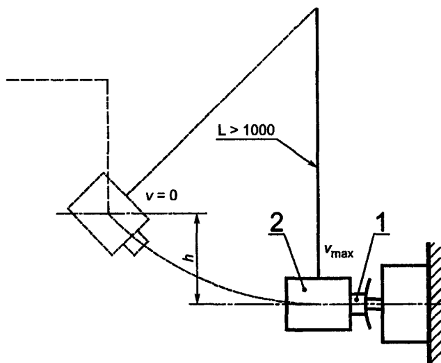
1 — деталь из резины с твердостью по Shore 45, диаметром 20 мм и длиной 18,5 мм; 2 — боек массой 1,6 кг
