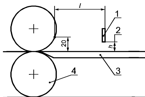
l — барьер; 2 — загрузочное отверстие; 3 — загрузочный стол; 4 — каток
