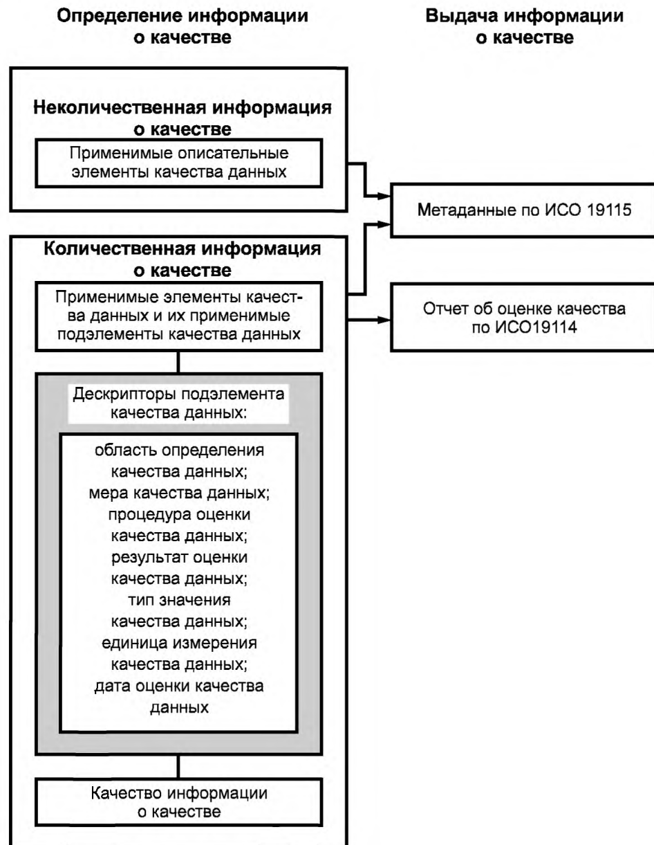
Рисунок 1 — Организация информации о качестве данных
