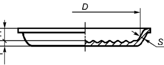
Рисунок 7 — Сковорода-гриль
