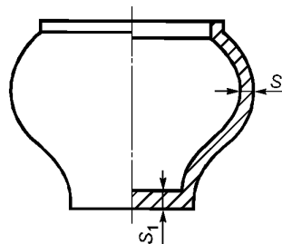
Рисунок 2 — Горшок
