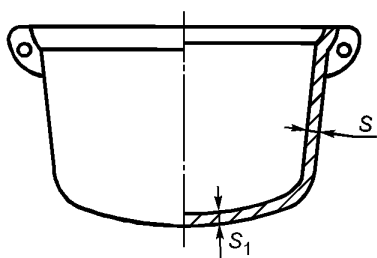
Рисунок 1 — Котел
