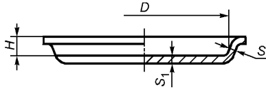
Рисунок 5 — Сковорода
