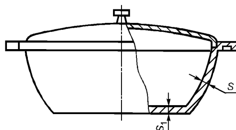
Рисунок 4 — Утятница/Гусятница
