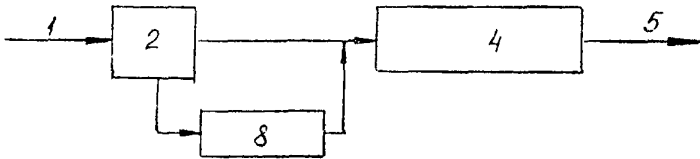
Рис. I. Принципиальные схемы разделения дождевого стока перед очистными сооружениями:
