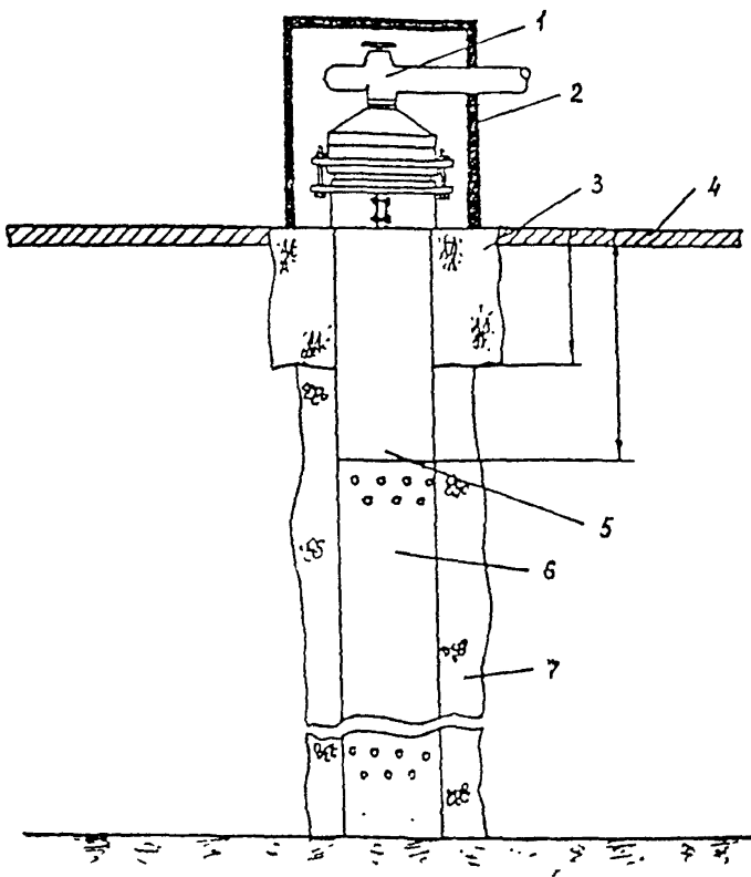
Рис. 4. Конструкция газовой скважины (для закрытых полигонов): 1 - оголовок скважины; 2 - колодез; 3 - бетон; 4 - изоляционный слой; 5 - обсадная труба без перфорации; 6 - перфорированная обсадная труба; 7 - щебень крупных фракций
