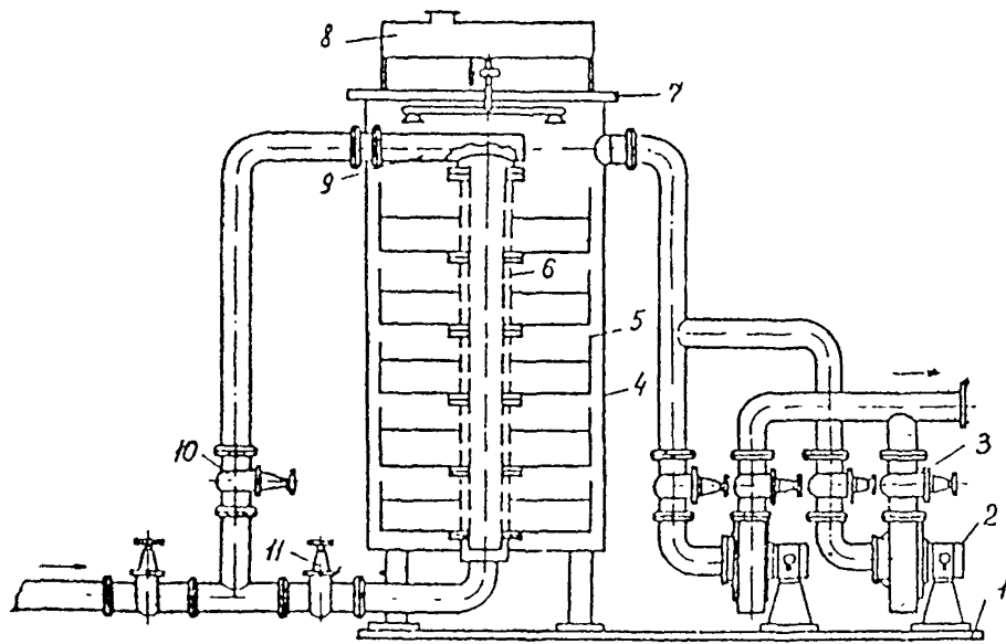
Рис. 3. Аппарат по очистке и осушке биогаза: 1 - рама; 2 - вентилятор; 3, 10, 11 - задвижки; 4 - корпус; 5 - контей- нер; 6 - ствол; 7 - крышка; 8 - бак; 9 - трубопровод
