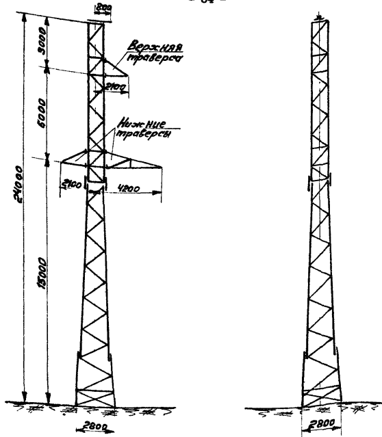
Техническая характеристика опоры
