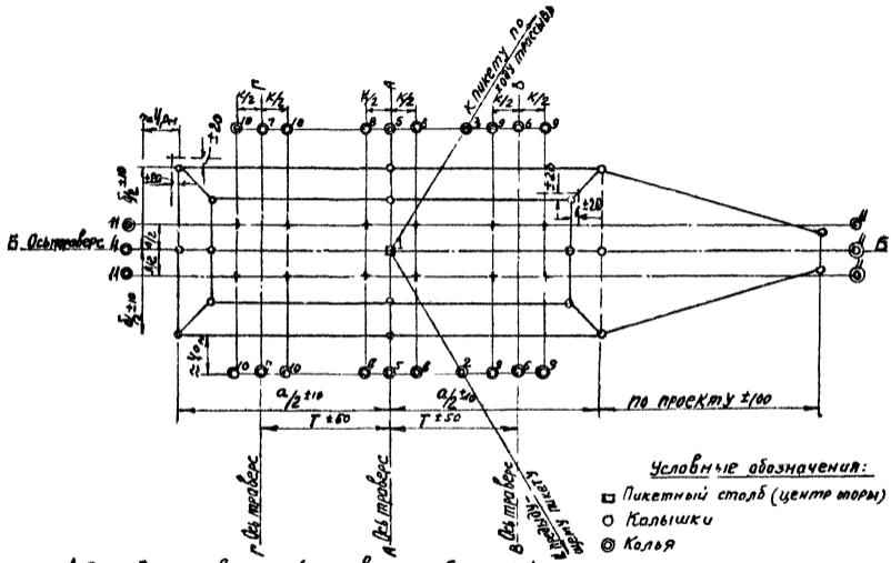
Рис.10 Допускаемые отклонения при разбивке котлована
