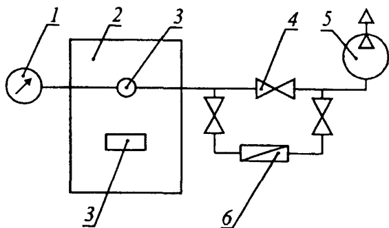
Рисунок 1 — Схема проверки камина на герметичность
