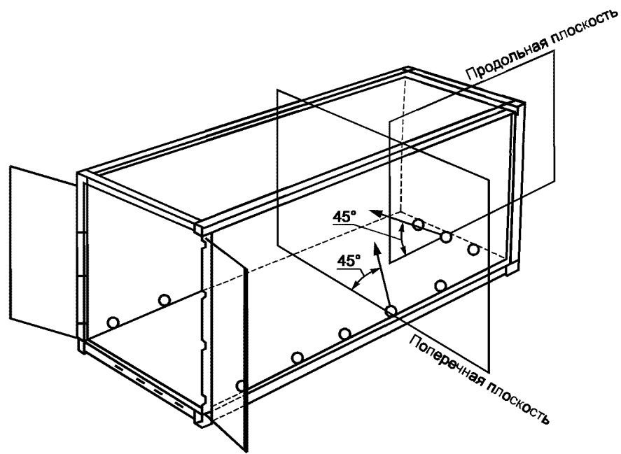
Рисунок Д.1 — Схемы приложения испытательных сил
