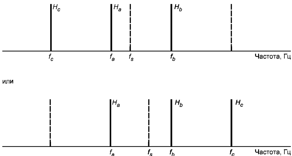
Рисунок Ж.1 — Примеры выбора частоты H_c
