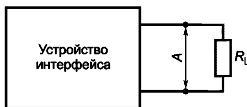
Рисунок 14 — Схема измерения выходных характеристик устройства интерфейса
