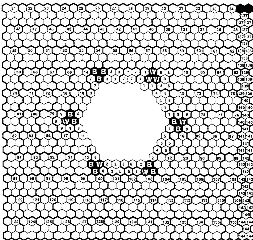
Рисунок 4 — Последовательность знаков символа MaxiCode
