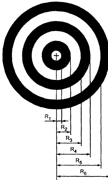
Рисунок 9 — Размеры шаблона поиска MaxiCode
