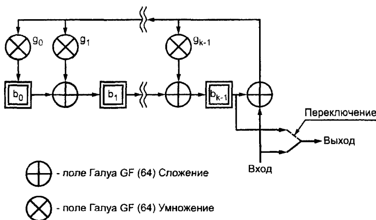
Рисунок 7 — Схема кодирования кодовых слов коррекции ошибок
