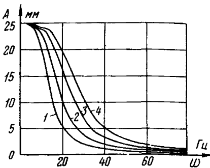
Рис. П.5. Зависимость влияния тяжения на угол вибрации провода марки АС 240/40:
