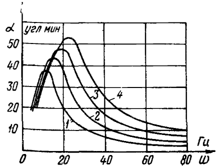
Рис. П.4. Зависимость влияния тяжения на амплитуду в пучности полуволн колебаний провода марки АС 240/40:
