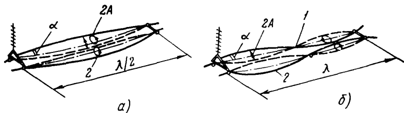
Рис.12.1. Формы колебаний проводов в подпролетах: a - с одной полуволной на подпролет; b - с двумя полуволнами на подпролет; 1 - узел колебаний; 2 - пучность колебаний; \lambda - длина волны колебаний; A - амплитуда колебаний; \alpha - угол колебаний в подпролетах; 0 - траектория движения провода в пучности волны колебаний
