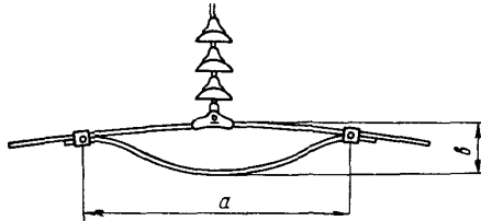
Рис.3.1. Петлевой гаситель вибрации
