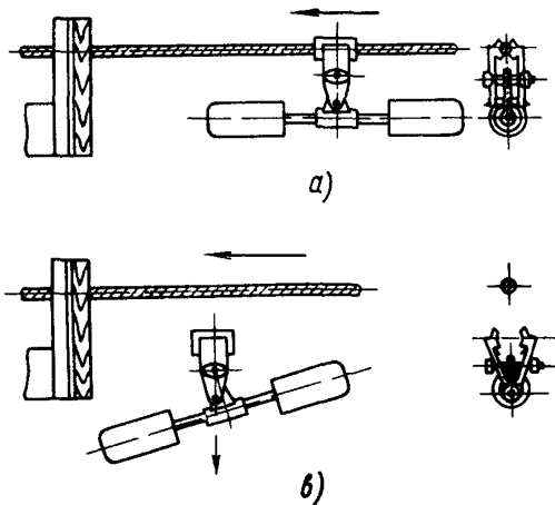
Рис.4.1. Схема расположения гасителей вибрации в переходных пролетах длиной до 500 м
