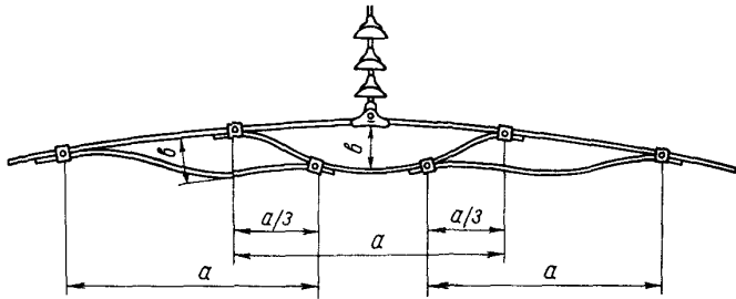
Рис.3.2. Трехпетлевой гаситель вибрации
