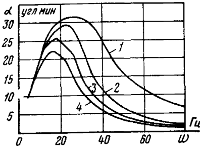
Рис. П.3. Зависимость угла вибрации провода от интенсивности турбулентности воздушного потока ( I_t ): 1 - ламинарный поток; 2 - I_t = 5\% ; 3 - I_t = 10\% ; 4 - I_t = 15\%
