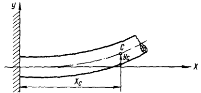
Рис.2.2. Деформированное состояние провода при жестком закреплении на конце: y_c - изгибная амплитуда; x_c - расстояние от последней точки контакта провода с зажимом
