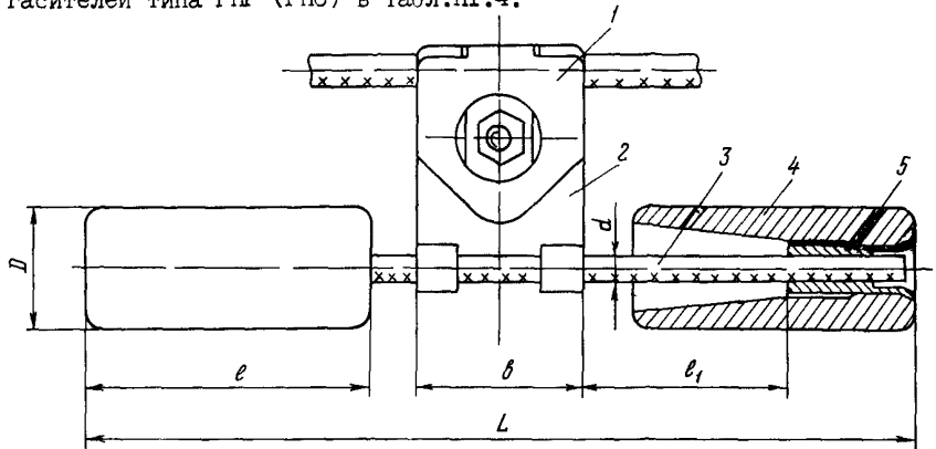
Рис. III.6. Конструкция гасителей вибрации типа ГВН (усовершенствованный), ГПГ:
