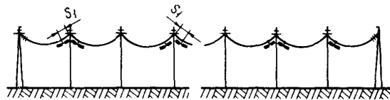
Рис.3.3. Схема установки гасителей вибрации на ВЛ: a - установка гасителей с обеих сторон пролета; b - установка гасителей с одной стороны пролета
