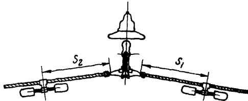
Рис.3.4. Расположение гасителей вибрации у поддерживающего зажима
