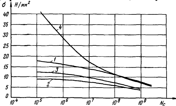
Рис. III.2. Кривые накопленных за год напряжений для провода АС 560/50: 1 - испытания проведены на ровной открытой местности, \sigma_{\text{стат}} = 0,2\sigma_B ( \sigma_B - предел прочности провода на разрыв); 2 - испытания проведены на холмистой местности, \sigma_{\text{стат}} = 0,2\sigma_B ; 3 - испытания проведены на холмистой местности, \sigma_{\text{стат}} = 0,27\sigma_B ; 4 - пограничная кривая СИПЭ
