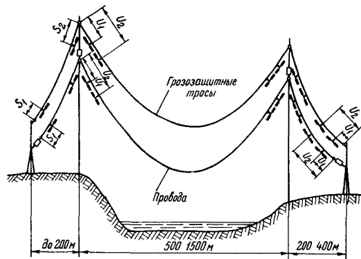
Рис.4.2. Схема расположения гасителей вибрации в переходных пролетах длиной до 1500 м
