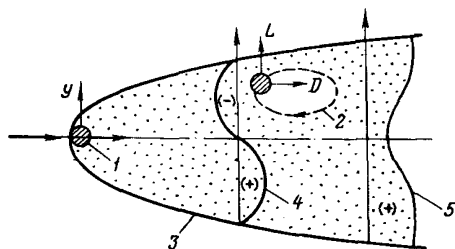
Рис.12.3. Аэродинамические силы, действующие на подветренный провод: L - подъемная сила; D - сила лобового сопротивления; 1 - наветренный провод; 2 - траектория движения подветренного провода; 3 - граница аэродинамического следа; 4 - эпюра подъемной силы в сечении следа; 5 - эпюра лобового сопротивления в сечении следа
