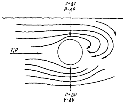
Рис.2.3. Схема вихреобразования за проводом
