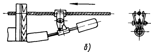
Рис.4.2. Схема расположения гасителей вибрации в переходных пролетах длиной до 1500 м
