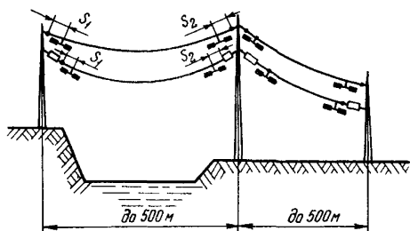
Рис.4.1. Схема расположения гасителей вибрации в переходных пролетах длиной до 500 м
