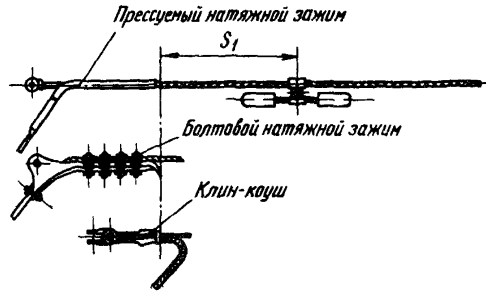
Рис.3.5. Расположение гасителя вибрации у натяжных зажимов
