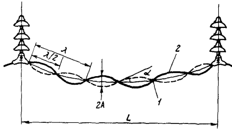
Рис.2.1. Стоячая волна вибрации провода в пролете ВЛ; 1 - узел колебаний; 2 - пучность; L - длина пролета; \lambda - длина волны колебаний; A - амплитуда колебаний; 2A - размах колебаний; \alpha - угол вибрации
