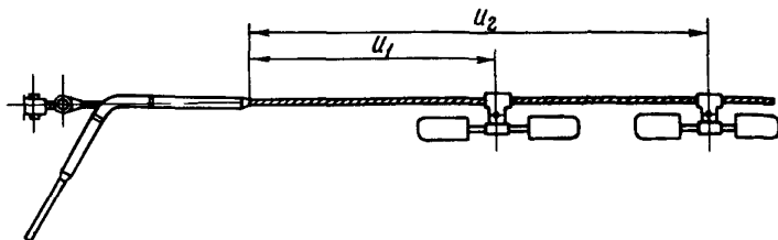
Рис.4.4. Расположение двух гасителей вибрации у натяжного зажима в переходном пролете длиной 500-1500 м
