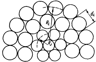
Рис. III.1. Поперечное сечение многоповивного сталеалюминиевого провода
