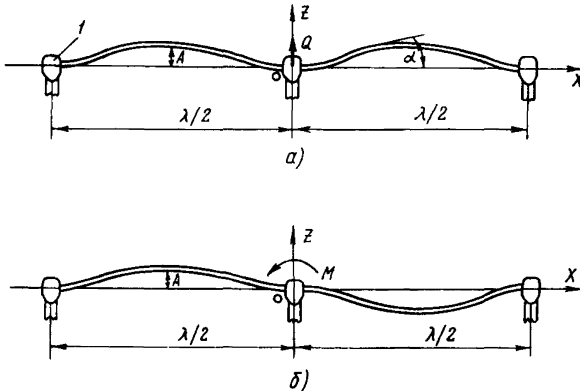
Рис. П2.5. Формы субколебаний провода:
