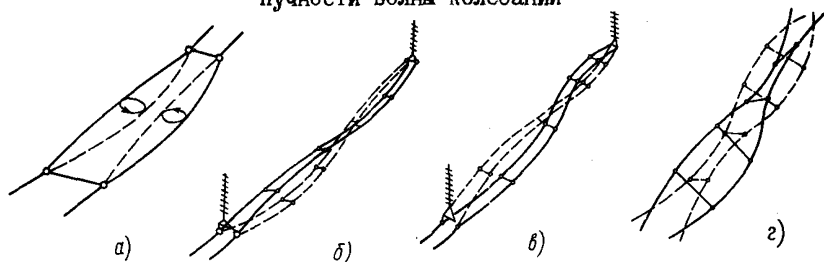
Рис.12.2. Виды колебаний проводов, вызываемых воздействием аэродинамического следа: a - колебания проводов в подпролетах; b - вертикальные колебания; б - горизонтальные колебания; z - крутильные колебания
