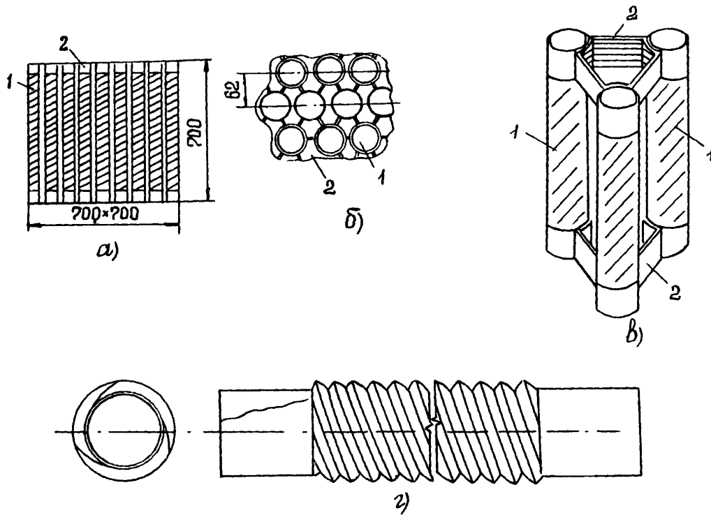
Рис. 18. Трубчатый ороситель ТГ44: а — блок оросителя; б — фрагмент блока оросителя (план); в — фрагмент блока оросителя (аксонометрия); з — элемент оросителя; 1 — гофрированная трубка; 2 — дистанционная фигурная втулка
