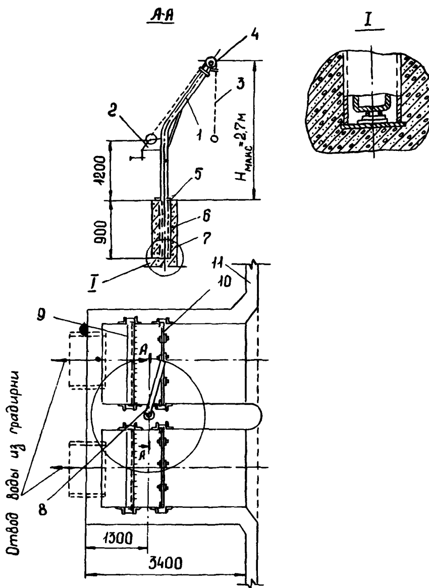
Рис. 1. Ручной поворотный кран:
