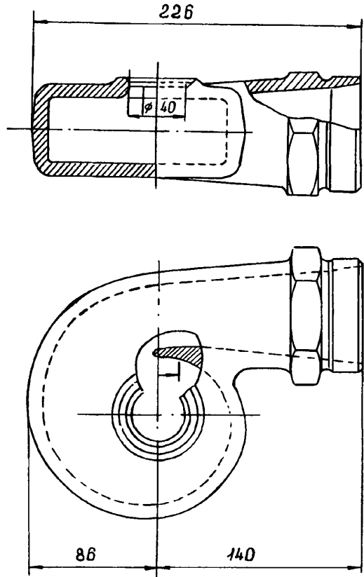
Рис. 6. Эвольвентное промывочное сопло диаметром 40 мм
