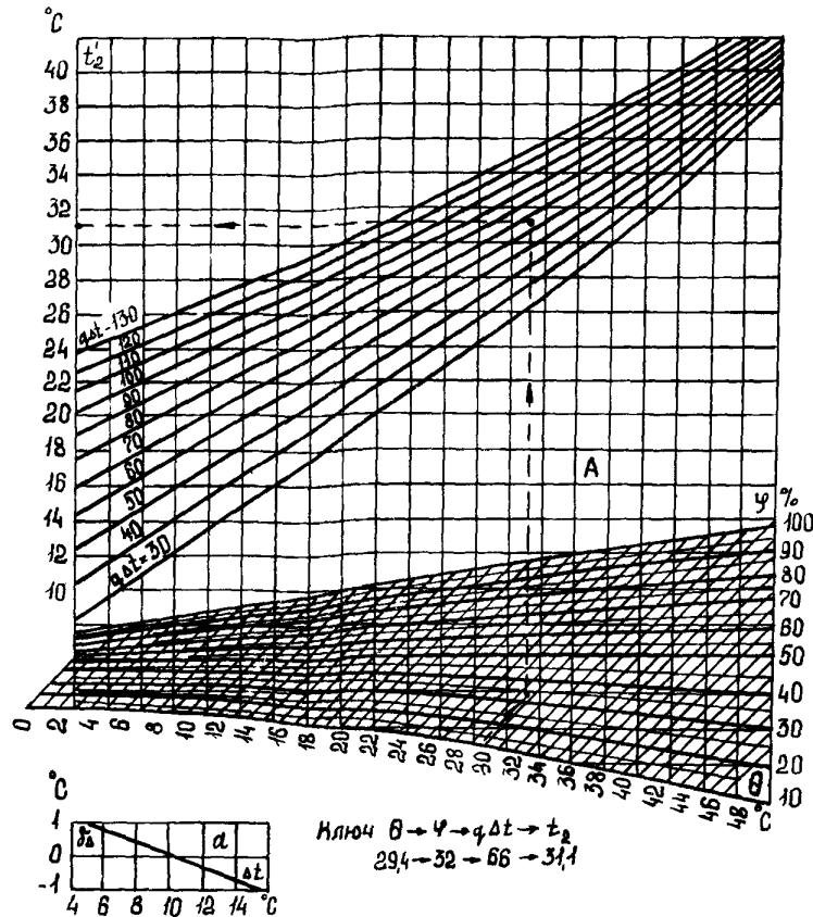
Рис. П4.1. Нормативная характеристика башенной градирни площадью орошения 4200 м 2 с двухъярусным оросителем высотой 2,85 м и расстоянием в свету между асбестоцементными листами 25 мм. Высота вытяжной башни — 100 м, воздухоподводящего окна — 5,5 м. градирня с водоуловителем
