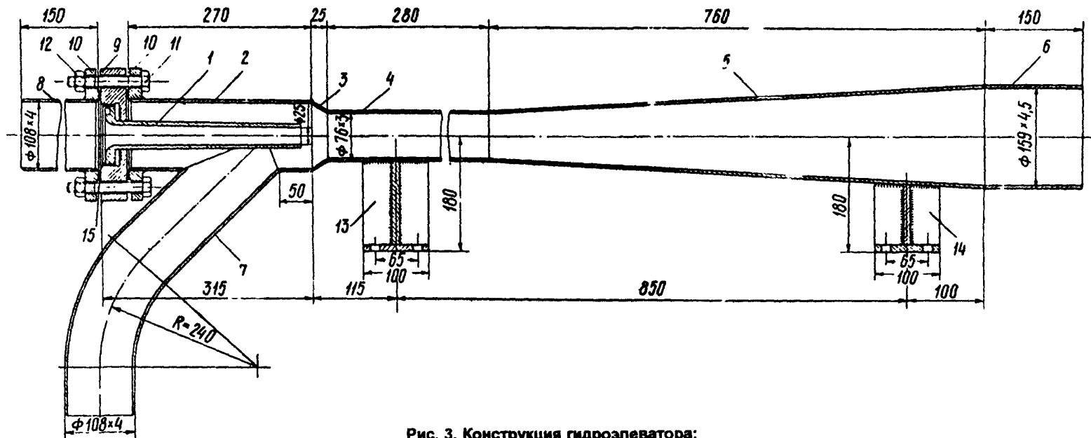
Рис. 3. Конструкция гидролеватора:
