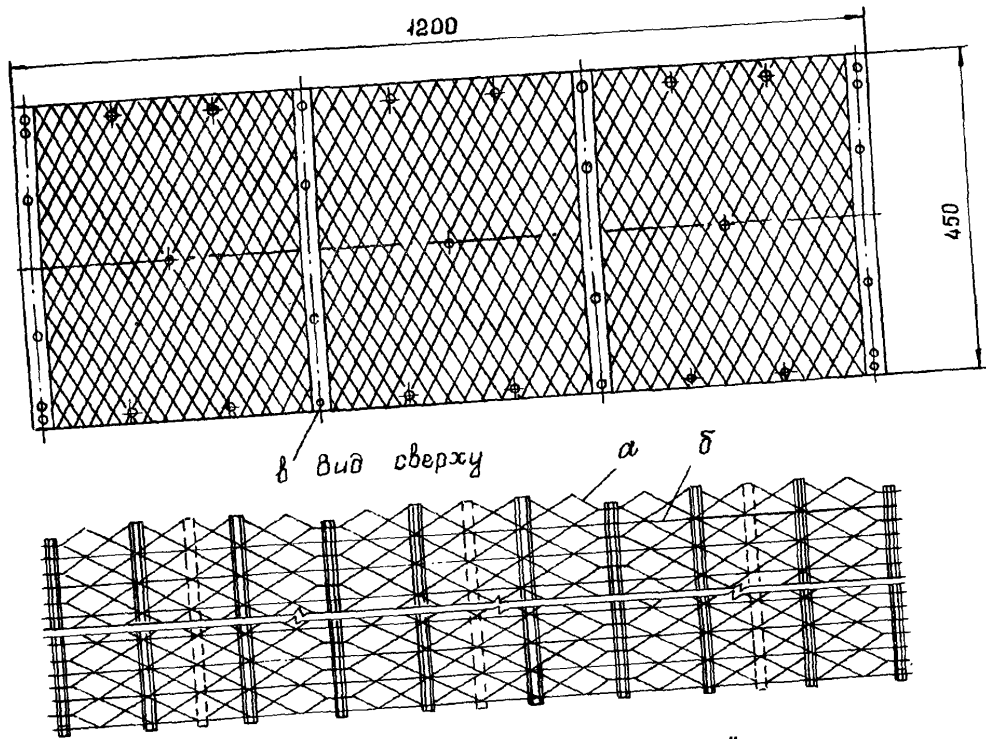
Рис. 15. Пластмассовый блок "Бальке-Дюрр": а — волнистая решетка; б — плоская решетка; в — втулка
