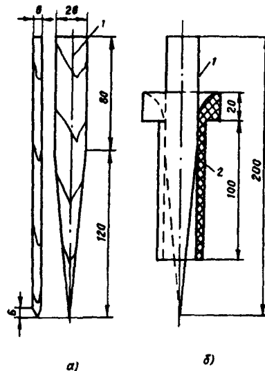
Рис. 5. Клин для изменения расхода воды через насадок диаметром 25 мм: а — конструкция клина; б — установка клина в насадке; 1 — деревянный клин; 2 — сливной насадок
