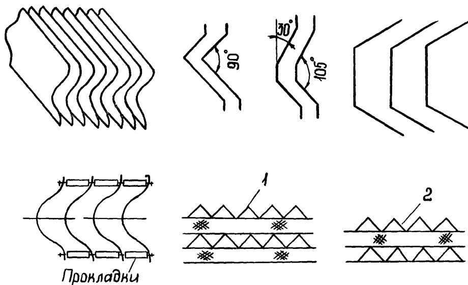
Рис. 20. Профили элементов пластмассовых водоуловителей:
