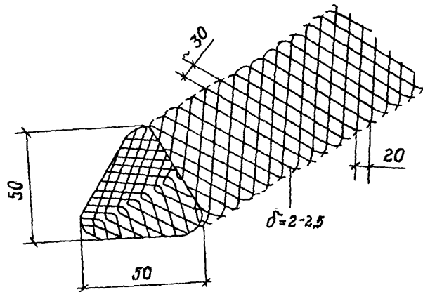
Рис. 16. Решетчатая призма ПР-50
