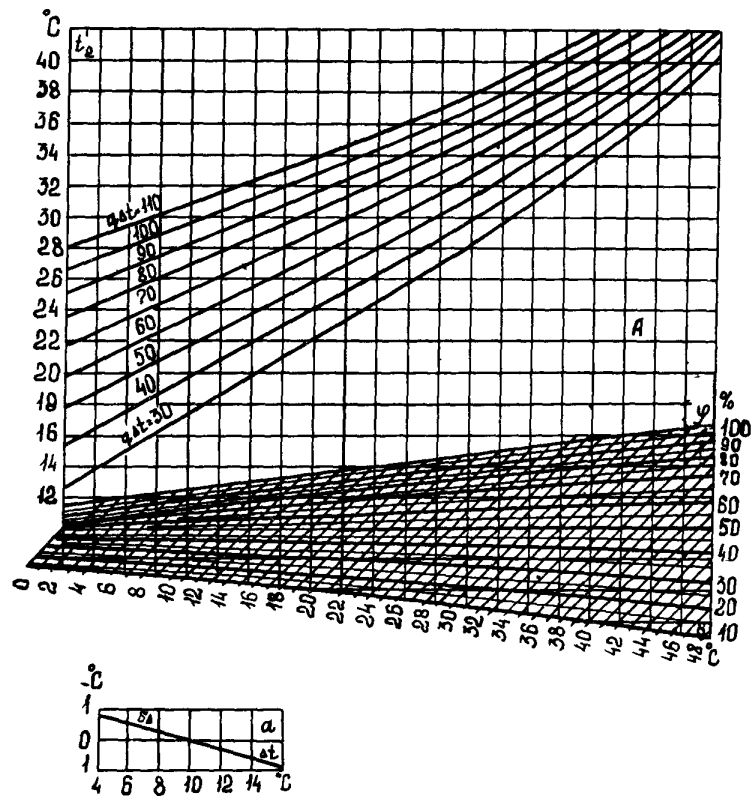
Рис. П4.9. Нормативная характеристика башенной градирни площадью орошения 1200 м 2 без водоуловителя, с лотковым водораспределением, с двухъярусным оросителем высотой 3,2 м и расстоянием в свету между асбестоцементными листами 25 мм. Высота вытяжной башни — 49,5 м, воздухопроводных окон — 3,55 м
