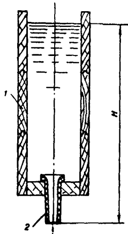
Рис. 4. Установка сливных насадков в рабочих лотках: 1 — лоток, 2 — насадок; H — расчетный напор воды перед насадком, м вод.ст.
