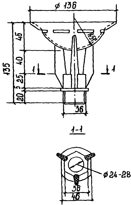
Рис. 10. Отражательное сопло с перфорированным отражателем
