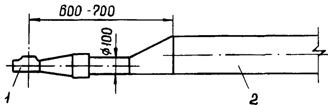
Рис. 7. Крепление концевго промывочного эвольвентного сопла на трубопроводе:
