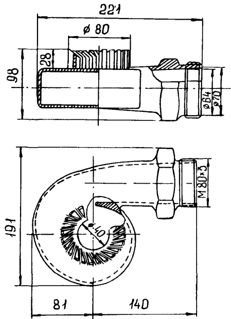
Рис. 13. Центробежное разбрызгивающее сопло с рассекателем водяного факела
