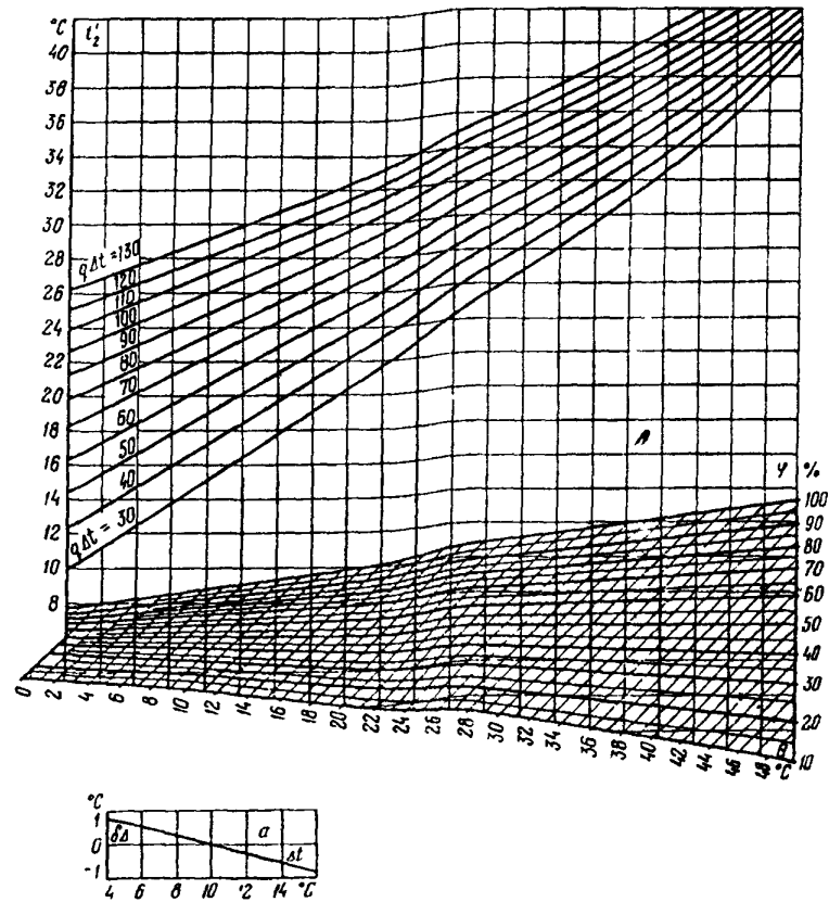
Рис. П4.4. Нормативная характеристика башенной грядирни: площадью орошения 3200 м 2 с двухъярусным оросителем высотой 2,65 м и расстоянием в свету между асбестоцементными листами 24 мм Высота вытяжной башни — 82 м, воздухоходного окна — 5,0 м, грядирня с водоуловителем, площадью орошения 1600 м 2 без водоуловителя при расстоянии в свету между асбестоцементными листами 32 мм и высоте оросителя 2,4 м Высота вытяжной башни — 54,10 м, воздухоходного окна — 3,55 м
