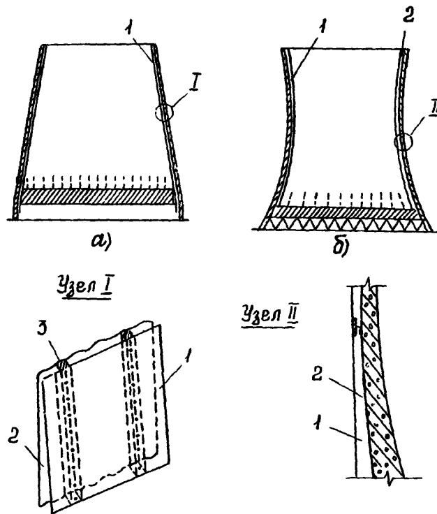
Рис. 21. Вытяжная башня градирни с защитным экраном: а — железобетонная башня; б — каркасно-обшивная башня; 1 — защитный экран, 2 — вентилируемый зазор, 3 — деревянный, антисептированный брус, фиксирующий значение вентилируемого зазора
