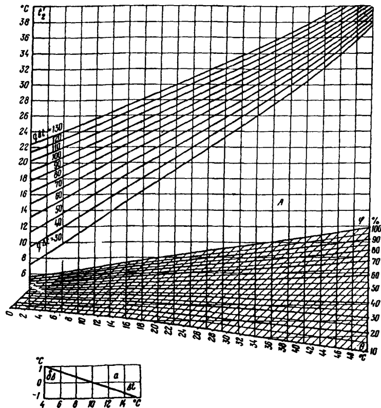
Рис. П4.3. Нормативная характеристика башенной грядирни площадью орошения 4000 м 2 с двухъярусным оросителем высотой 2,52 м и расстоянием в свету между асбестоцементными листами 19 мм Высота вытяжной башни — 90 м, воздухоходного окна — 5,0 м, грядирня без водоуловителя
