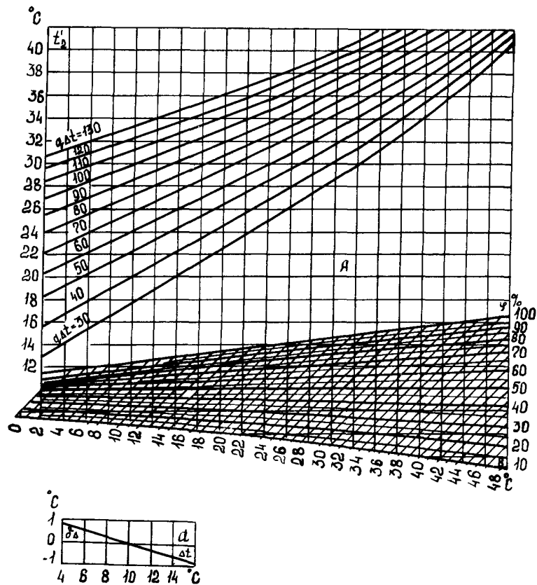
Рис. П4.8. Нормативная характеристика башенной градирни: площадь орошения 1600 м 2 без водоуловителя с лотковым водораспределением, с двухъярусным оросителем высотой 2,65 м и расстоянием в свету между асбестоцементными листами 20 мм Высота вытяжной башни — 54,1 м, воздухоходных окон — 3,55 м, площадь орошения 1600 м 2 без водоуловителя, с одноярусным оросителем высотой 2,44 м из деревянных блоков типа КП-90-160 Высота вытяжной башни — 53,76 м, воздухоходных окон — 3,3 м, площадь орошения 1200 м 2 без водоуловителя, с лотковым водораспределением, двухъярусным оросителем высотой 3,2 м и расстоянием в свету между асбестоцементными листами 25 мм Высота вытяжной башни — 49,5 м, воздухоходных окон — 3,55 м, площадь орошения 1200 м 2 без водоуловителя, с одноярусным оросителем высотой 2,65 м из деревянных блоков типа КПШ-48-200 Высота вытяжной башни — 48,4 м, воздухоходных окон — 3,3 м, площадь орошения 800 м 2 без водоуловителя, с одноярусным оросителем высотой 2,46 м из деревянных блоков типа КП 90-115 Высота вытяжной башни — 45 м, воздухоходных окон — 3,3 м
