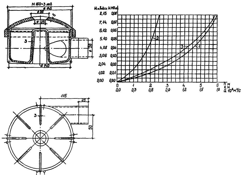
Рис. 9. Эвольвентное сопло для брызгальных градирен:
