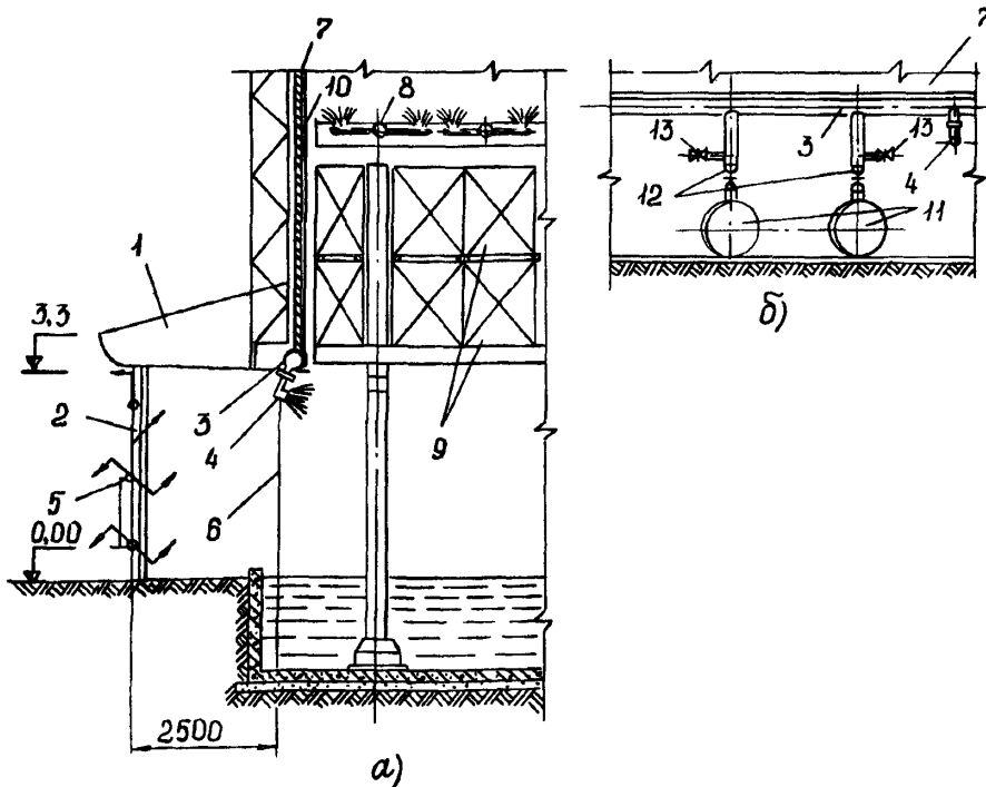
Рис. 22. Комбинированное противообледенительное устройство башенной градирни:
