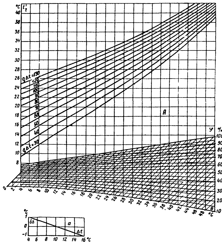
Рис. П4.10. Нормативная характеристика башенной градирни: площадью орошения 2100, 2600, 3200 и 4000 м 2 с водоуловителем, напорным водораспределением, одноярусным оросителем высотой 2,85 м из деревянных блоков типа КП-100-160, с расстоянием в свету между щитами 25 мм. Высота вытяжной башни соответственно 64,8 м, 71,0 м, 81,0 м и 90,0 м, высота воздухоходных окон соответственно 3,8 м, 4,3 м, 5,0 м, 5,5 м; площадью орошения 1500 м 2 с напорным водораспределением, двухъярусным оросителем высотой 3,0 м из деревянных блоков типа КПЯ-50х32 с ячейками 50х32 мм, а также высотой 2,6 м из деревянных блоков типа КПЯ-45х29 с ячейками 45х29 мм, железобетонной гиперболической башней высотой 55,3 м, воздухоходных окон — 3,4 м; площадью орошения 500 м 2 без водоуловителя, с одноярусным оросителем высотой 1,6 м из деревянных блоков типа ШЯ-48 с ячейками 48х48 мм. Высота вытяжной башни — 40,0 м, воздухоходных окон — 2,5 м
