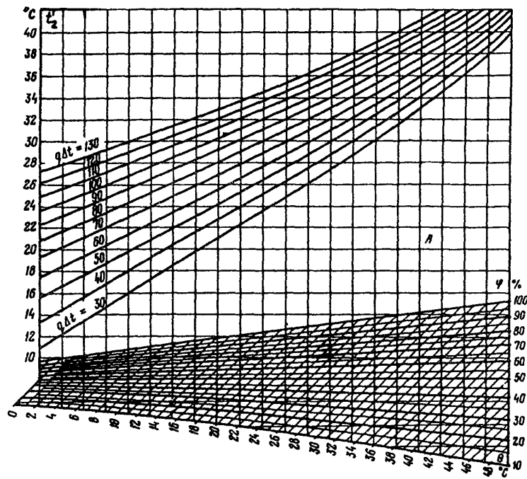
Рис. П4.5. Нормативная характеристика башенной градирни: площадью орошения 2100 м 2 с двухъярусным оросителем высотой 2,85 м и расстоянием в свету между асбестоцементными листами 25 мм. Высота вытяжной башни — 64,8 м, воздухоходного окна — 3,80 м, градирня с водоуловителем, площадью орошения 2600 м 2 с двухъярусным оросителем высотой 2,85 м и расстоянием в свету между асбестоцементными листами 25 мм. Высота вытяжной башни — 71,0 м, во- здухоходного окна — 4,30 м, градирня с водоуловителем
