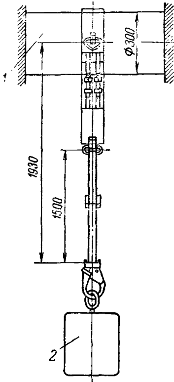
Рис. П.7.3. Схема испытательного устройства для статической нагрузки предохранительных поясов (размеры в миллиметрах):
