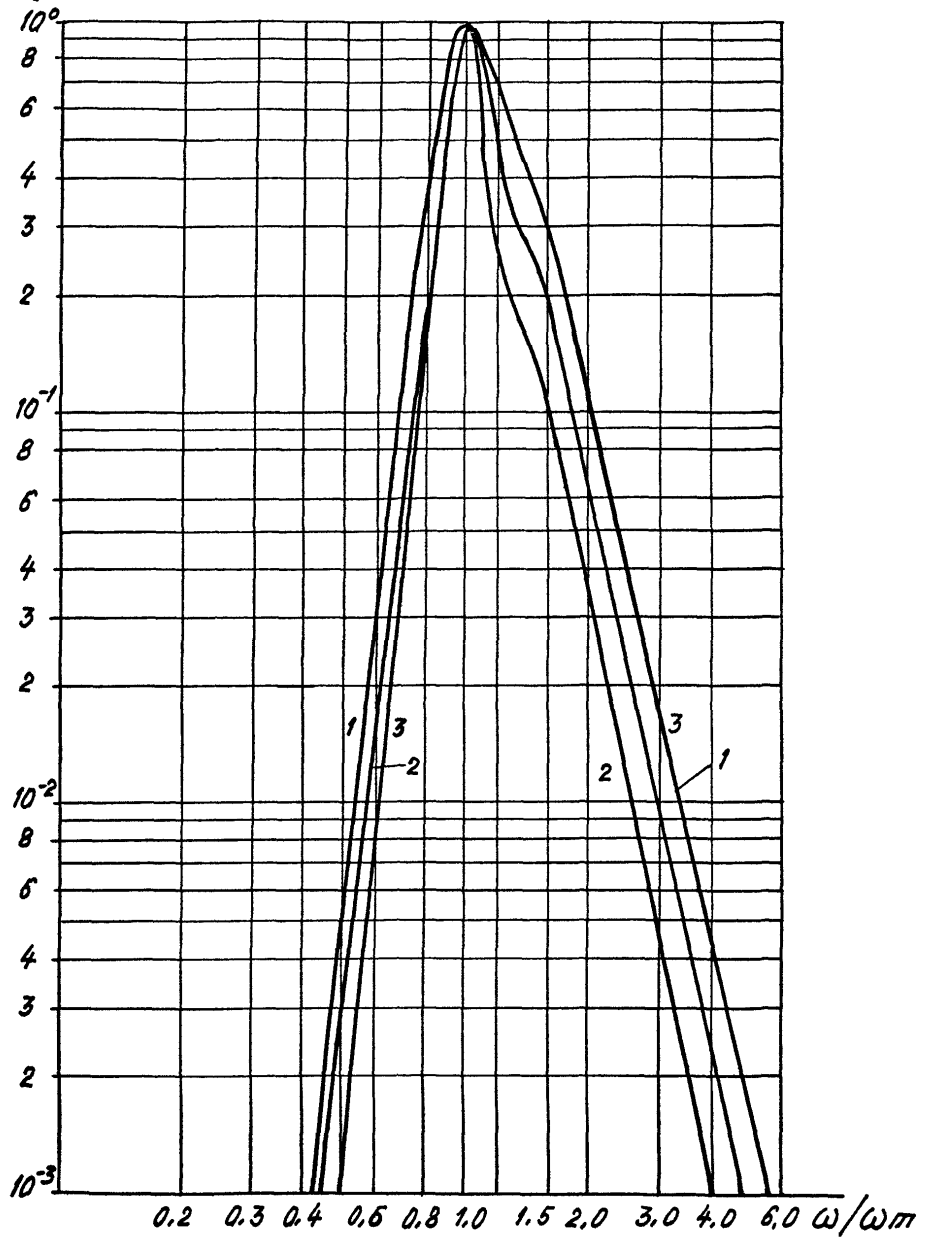
Рис.4. График зависимости безразмерной спектральной плотности S_f(\omega)/S_f(\omega_m) и величины n(\omega)/n(\omega_m) от безразмерной частоты \omega/\omega_m
