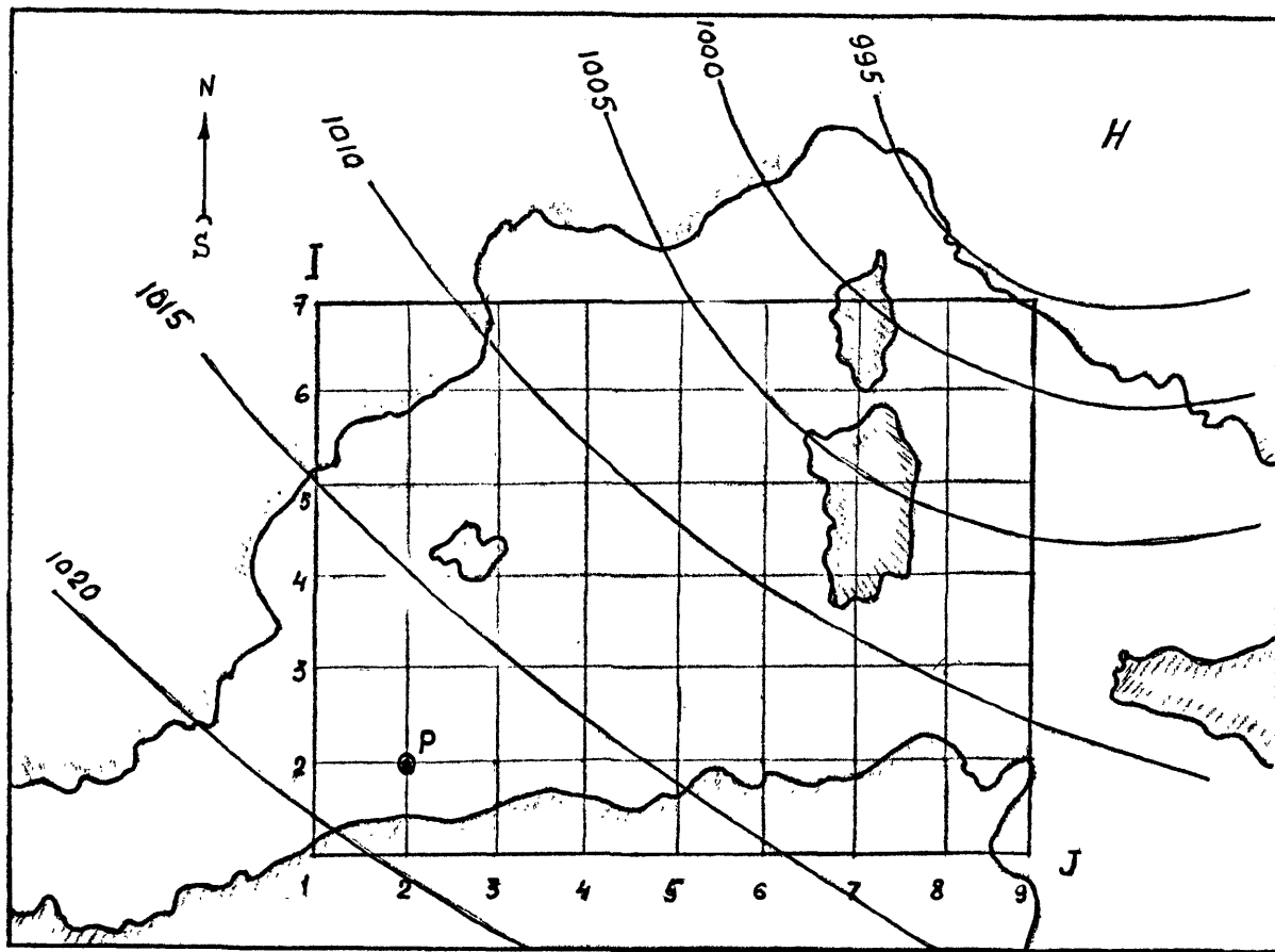
Рис. П 3. Схема к расчету элементов волн в точке P.
