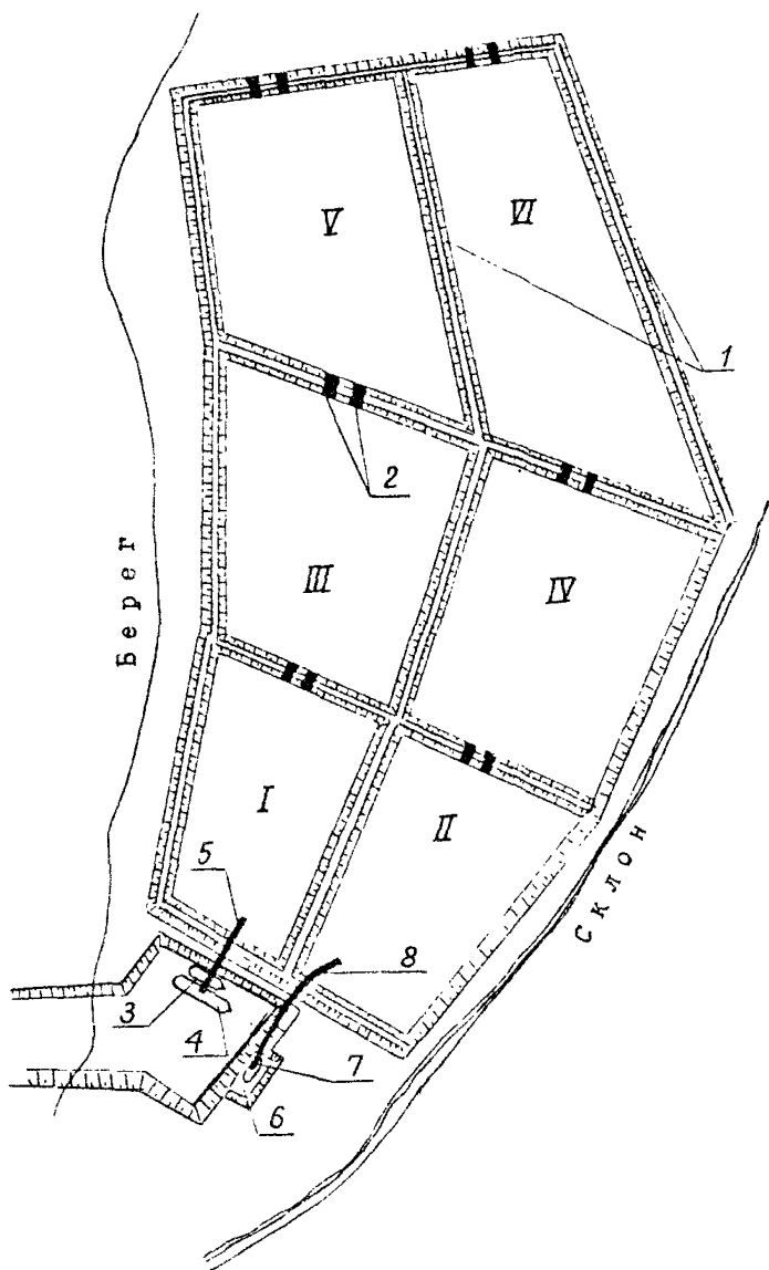
Рис. 4. Схема берегового отвала в порту Керчь: 1—У1 — карты намыва; 1 — дамбы обвалования; 2 — водопроводы; 3 — плавучий причал; 4 — самоотвозный землесос; 5 — береговой пульпопровод; 6 — депозит; 7 — шаландоперегрузатель; 8 — плавучий пульпопровод
