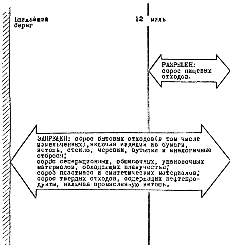
Рис.1 Ограничения и условия сброса мусора (в ОСОБЬЮ РАЙОНА) по "Международной конвенции по предотвращению загрязнения моря с судов 1973г." и в Балтийском море по "Конвенции по защите морской среды района Балтийского моря 1974г."
