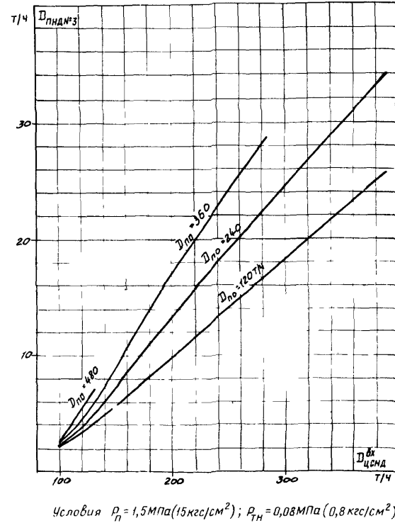
Рис.70 ТИПОВАЯ ЭНЕРГЕТИЧЕСКАЯ ХАРАКТЕРИСТИКА ТУРБОАГРЕГАТА ЗАВИСИМОСТЬ РАСХОДА ГРЕЮЩЕГО ПАРА ПНД № 3 ОТ РАСХОДА ПАРА НА ВХОДЕ В ЦСНД ПРИ ВОЗВРАТЕ КОНДЕНСАТА ПРОИЗВОДСТВЕННОГО ОТБОРА ПЕРЕД ПНД № 3 (ОДНОСТУПЕНЧАТЫЙ РЕЖИМ) Тип ПТ-135/165-130/15 ТМЗ
