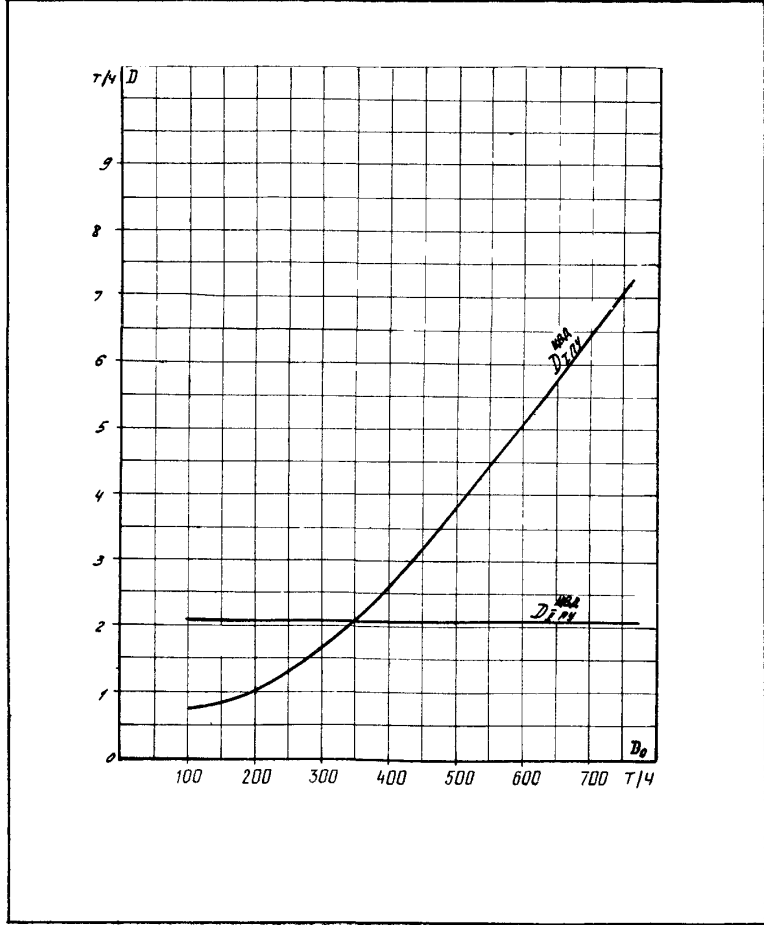
Рис.27 ТИПОВАЯ ЭНЕРГЕТИЧЕСКАЯ ХАРАКТЕРИСТИКА ТУРБОАГРЕГАТА ЗАВИСИМОСТЬ РАСХОДА ПАРА ОТ УПЛОТНЕНИЙ ЦВД ОТ РАСХОДА СВЕЖЕГО ПАРА Тип ПТ-135/165-130/15 ТМЗ
