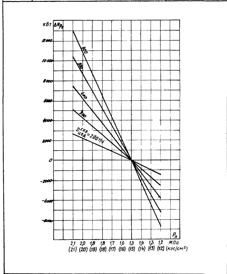
Рис.28 ТИПОВАЯ ЭНЕРГЕТИЧЕСКАЯ ХАРАКТЕРИСТИКА ТУРБОАГРЕГАТА ПОПРАВКИ К МОЩНОСТИ ЦВД НА ИЗМЕНЕНИЕ ДАВЛЕНИЯ В КАМЕРЕ ПРОИЗВОДСТВЕННОГО ОТБОРА Тип ПТ-135/165-130/15 ТМЗ
