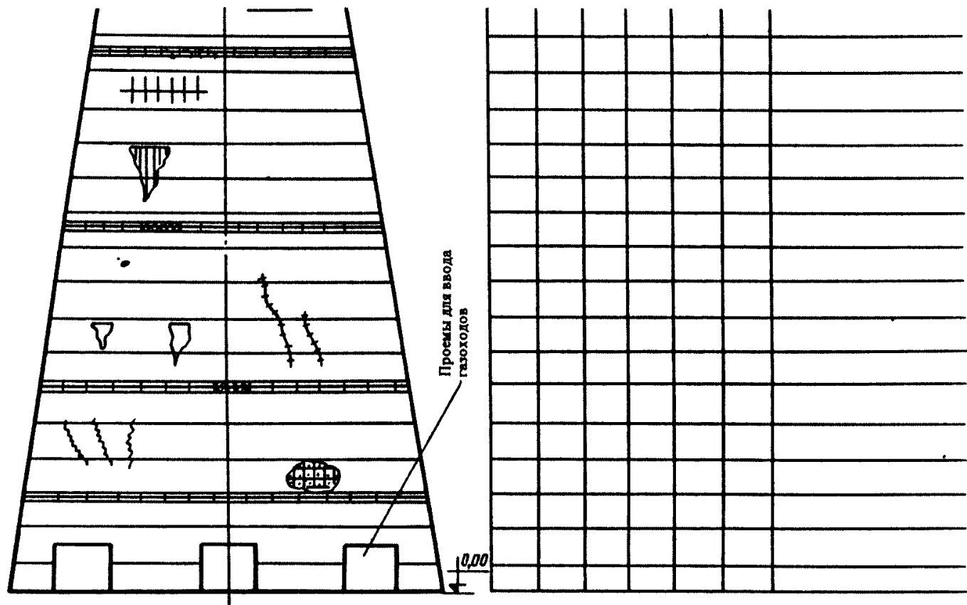
Рис. 3. Карта дефектов и результаты измерения прочности бетона железобетонной оболочки дымовой трубы
