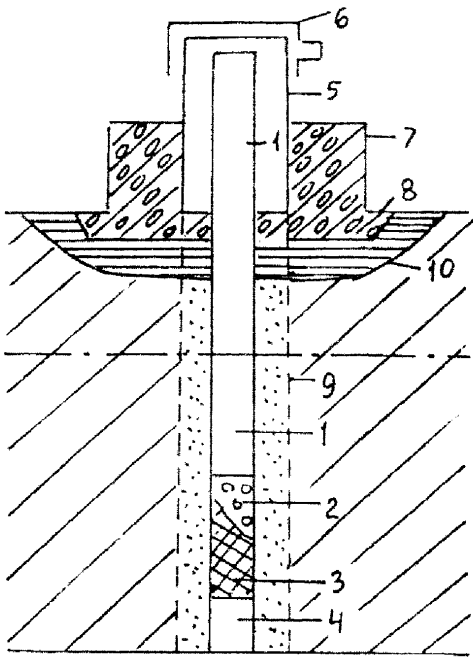
Рис. 3. Конструкция наблюдательной скважины:
