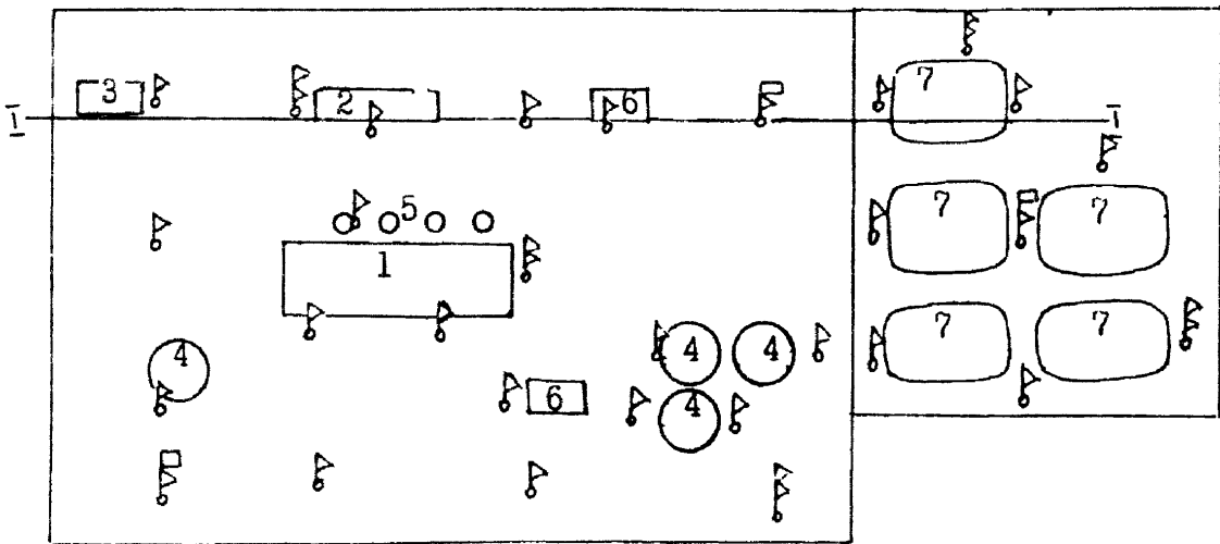
Рис. 1. План размещения скважин на промплощадке тепловой электростанции:
