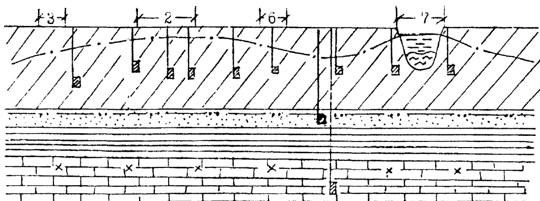
Рис. 2. Схематический геолого-гидрогеологический разрез I:
