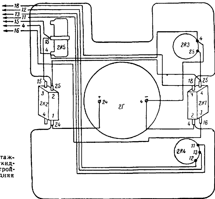
Рис. 1-6. Монтажная схема цоколя устройства У2.
