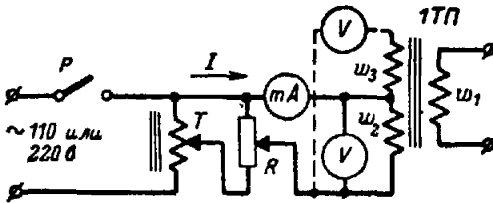
Рис. 2-5. Схема измерения сопротивлений холостого хода трансформатора 1ТП. P — рубильник; T — автотрансформатор; R — реостат; V — вольтметр; МА — миллиамперметр.
