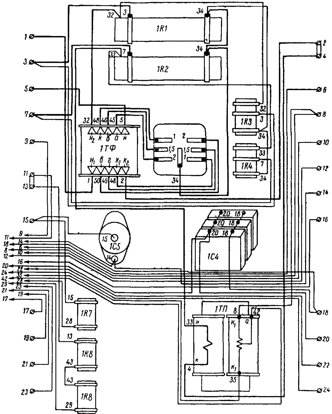
Рис. 1-3. Монтажная схема цоколя устройства VI.
