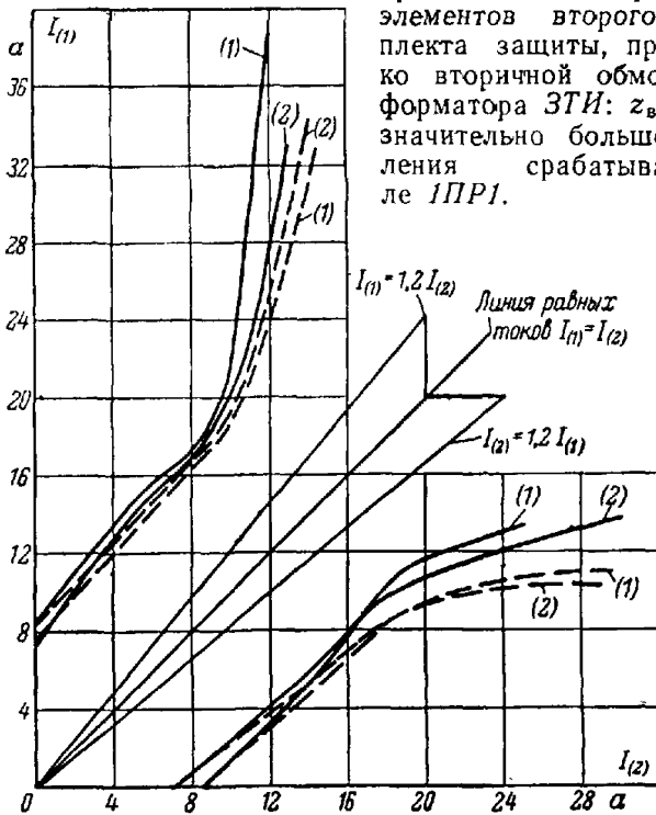
Рис. 1-19. Тормозные характеристики защиты; короткое замыкание ВО; h = 2 ; k = -10 ; R_{ПР} = 0 ; C_{ПР} = 0 . — \varphi = 155^\circ ; - - - \varphi = 205^\circ ;
