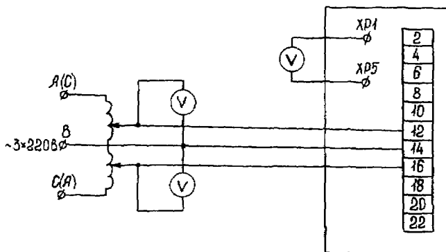
Рис. 4. Схема для испытания фильтра обратной последовательности
