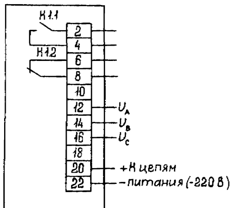
Рис. 1. Схема подключения реле
