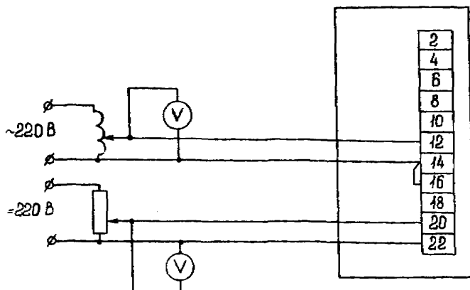
Рис. 3. Схема испытаний реле
