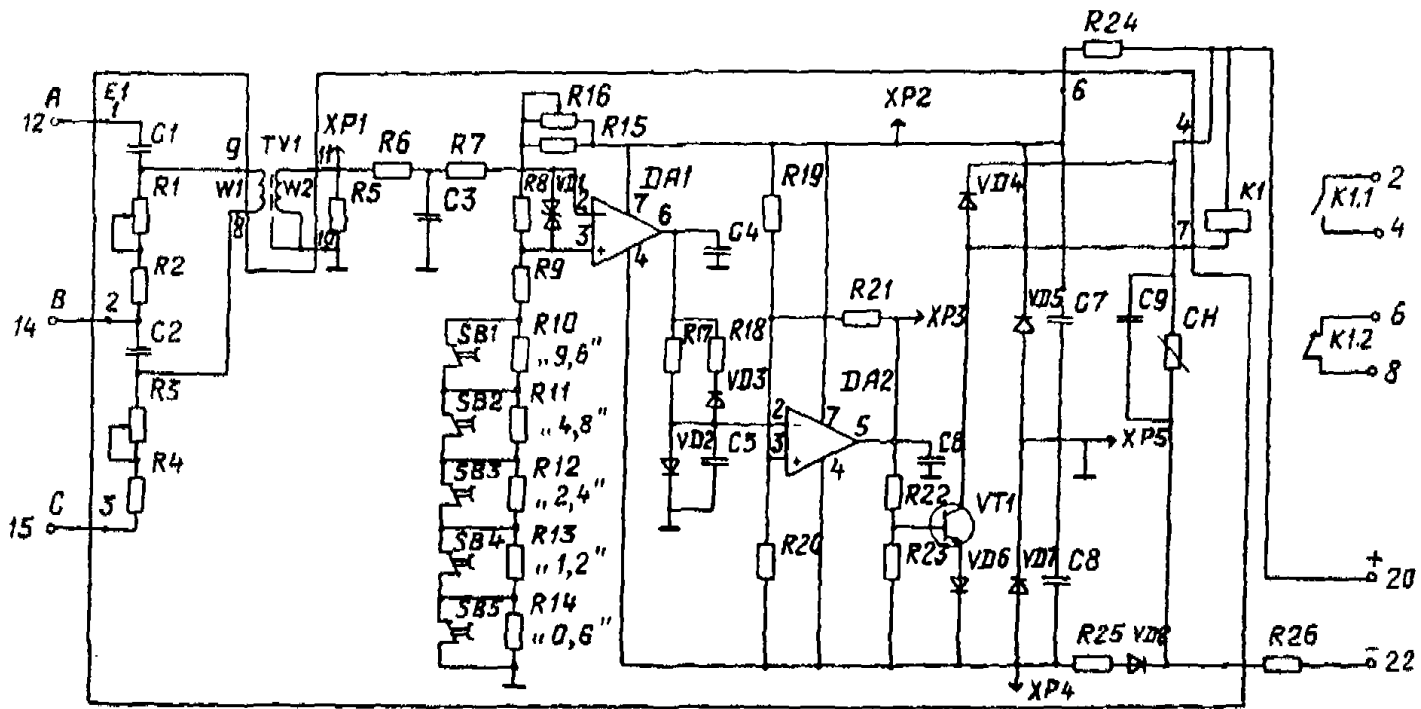
Рис. 2. Принципиальная схема реле
