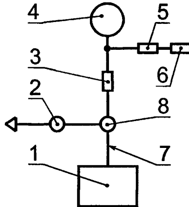
1 — аппарат ИВЛ; 2 — проверяемое устройство для измерения объема; 3 — сопротивление; 4 — модель легких; 5 — датчик давления; 6 — устройство для записи давления как функции времени с точностью \pm 2\% ; 7 — дыхательный контур; 8 — клапан выдоха
