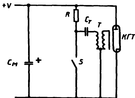
C_M — конденсатор-накопитель; C_T — триггерный конденсатор; KГТ — ксеноновая газоразрядная трубка; S — синхронный выключатель; R — резистор; T — триггерный трансформатор
