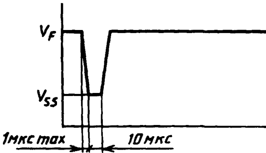
Рисунок 3 — Форма кривой изменения напряжения на выводах цепи поджига
