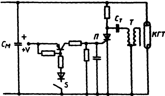
C_M — конденсатор-накопитель; C_T — триггерный конденсатор; КГТ — ксеноновая газоразрядная трубка; S — синхронный выключатель; \Pi — полупроводник; T — триггерный трансформатор
