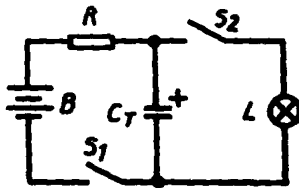
B — батарея; C_T — триггерный конденсатор; L — лампа-вспышка; S_1 — выключатель; S_2 — синхронный выключатель; R — резистор
