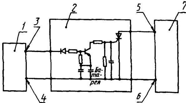
1 — фотоаппарат, 2 — адаптер, 3 — вывод синхронизатора с высоким потенциалом, 4 — вывод синхронизатора с низким потенциалом, 5 — вывод цепи поджига с высоким потенциалом, 6 — вывод цепи поджига с низким потенциалом, 7 — ИФО
