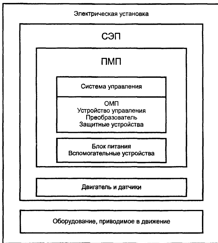
Рисунок 1 — Составные части электрической установки, включающей СЭП
