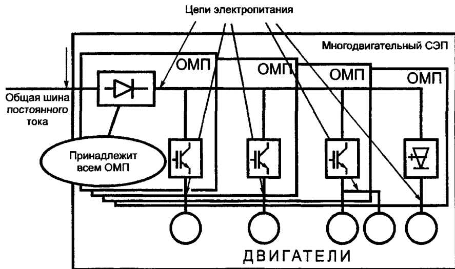
Рисунок 3 — Цели электропитания СЭП с общей шиной постоянного тока
