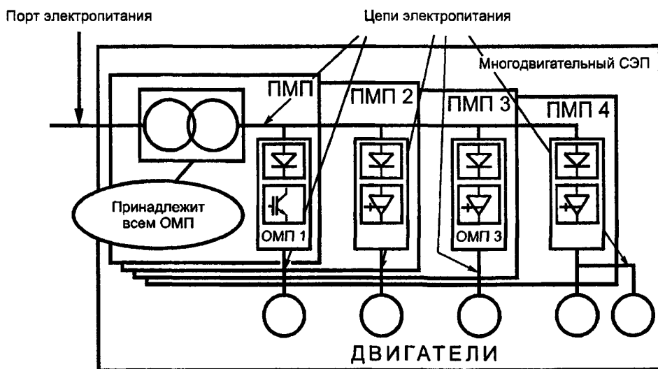
Рисунок 4 — Цели электропитания СЭП с общим входным трансформатором
