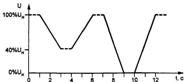
Рисунок 1 — Динамические изменения напряжения (провалы)
