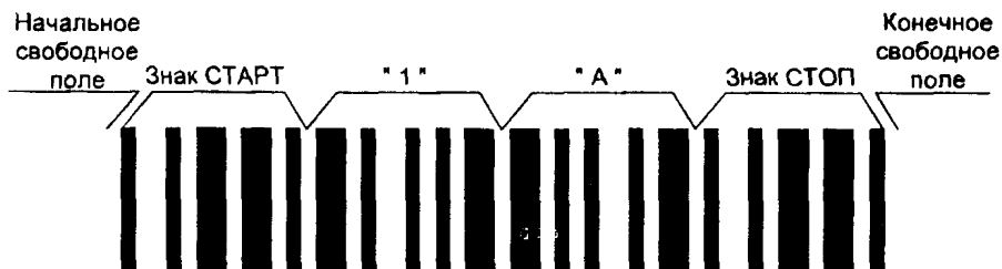
Рисунок 1 — Символ «Кода 39», в котором закодированы знаки «1А»
