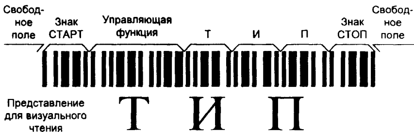
Рисунок Е.1 — Символ штрихового кода, в котором закодированы знаки ТИП
