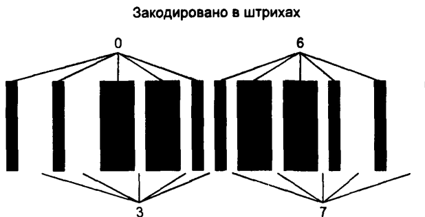
Рисунок 1 — Пары знаков символа “2 из 5 чередующийся”, кодирующие последовательность данных 03 67
