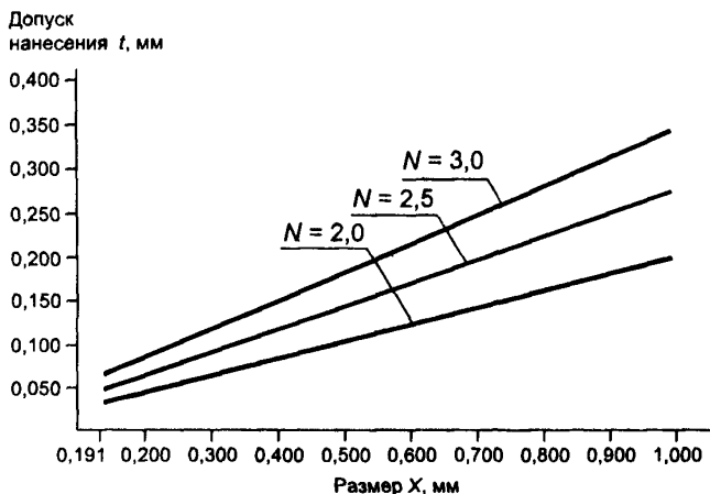
Рисунок 4 — Допуски для “2 из 5 чередующийся”
