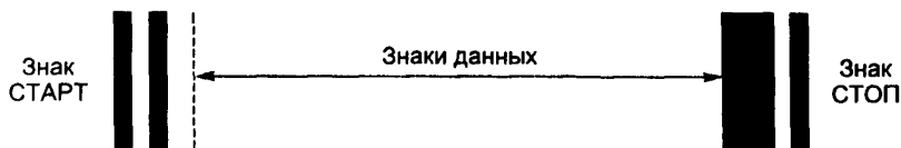
Рисунок 2 — Знаки СТАРТ и СТОП
