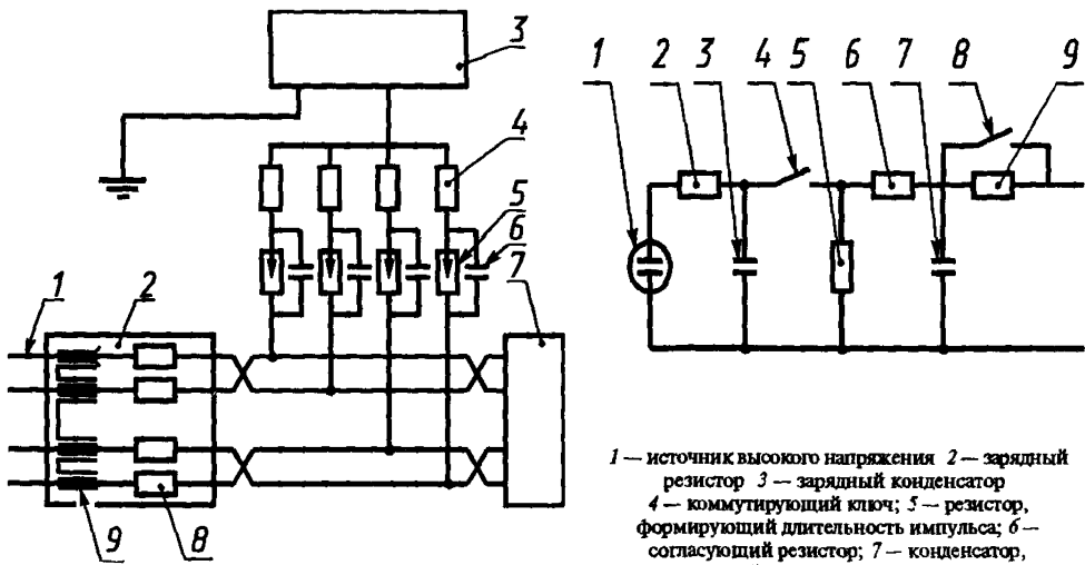
1 — провода линии связи; 2 — цепь развязки; 3 — ИГ; 4 — сопротивление в цепи связи; 5 — разрядник; 6 — конденсатор в цепи связи; 7 — испытуемое ТС; 8 — активное сопротивление катушки индуктивности; 9 — индуктивность 20 \text{ мГн}
