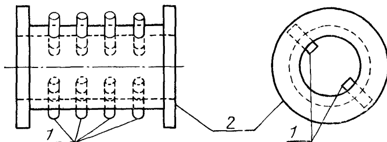
1 - подстроечные винты; 2 - круглый волновод
