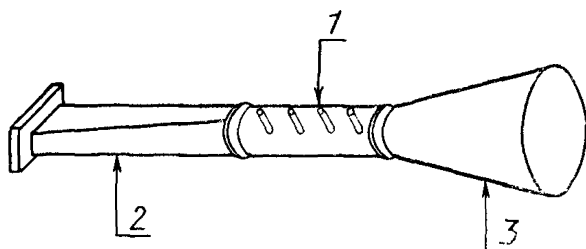
1 - круговой поляризатор, 2 - переход с прямоугольного на круглый волновод; 3 - конический рупор
