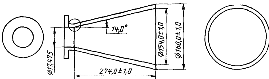
Рисунок В2 — Основные размеры рупорного облучателя
