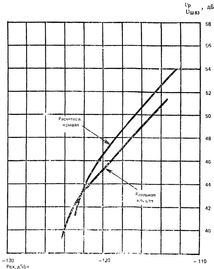
Рисунок 11 — Зависимость отношения сигнал/шум на выходе установки от уровня сигнала на входе
