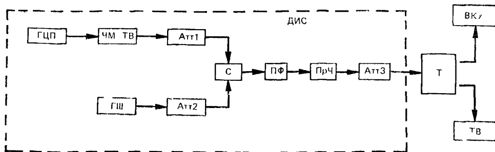
Рисунок 10 — Структурная схема измерения «динамического порога»
