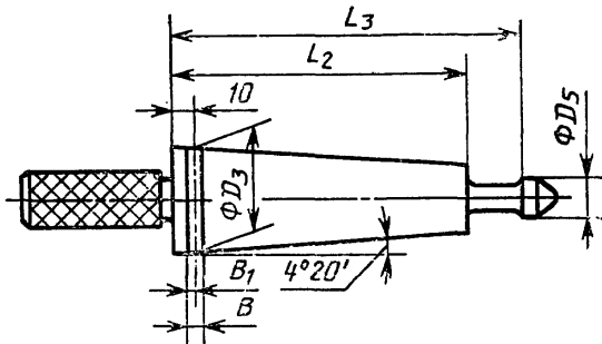
Калибр для патрона с закатанным торцом
