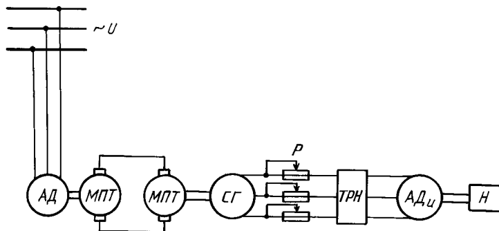
АД — асинхронный двигатель; МПТ — машины постоянного тока; СГ — синхронный генератор; АД—МПТ—СГ — система генератор—двигатель; Р — резистор; ТРН — тиристорный регулятор напряжения с фазным регулированием; АД н — испытываемый асинхронный двигатель; Н — нагрузка на валу асинхронного двигателя
