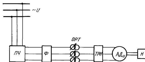
ПЧ — преобразователь частоты (статический или тиристорный); Ф — фильтр; ОРТ — однофазные регулировочные трансформаторы; ТРН — тиристорный регулятор напряжения с фазным управлением; АД н — испытываемый асинхронный двигатель; Н — нагрузка на валу асинхронного двигателя
