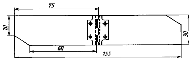
Рисунок 2 — Давяльная пластинка
