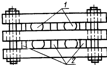
1—образцы, 2—ограничители
