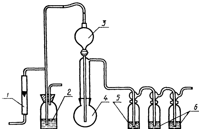
Аппарат для определения сульфидной серы
