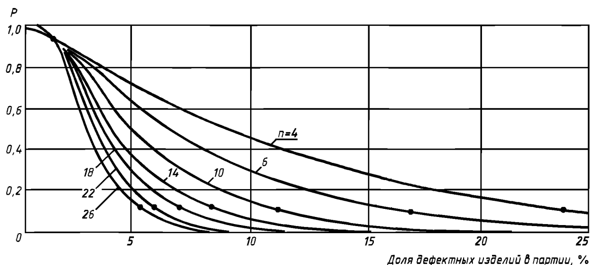
Р и с у н о к 4 — Кривые оперативных характеристик одноступенчатых планов контроля таблицы 9 для AQL = 1,5 \% : с установленным односторонним пределом для единичных значений и известным средним квадратическим отклонением 1)
