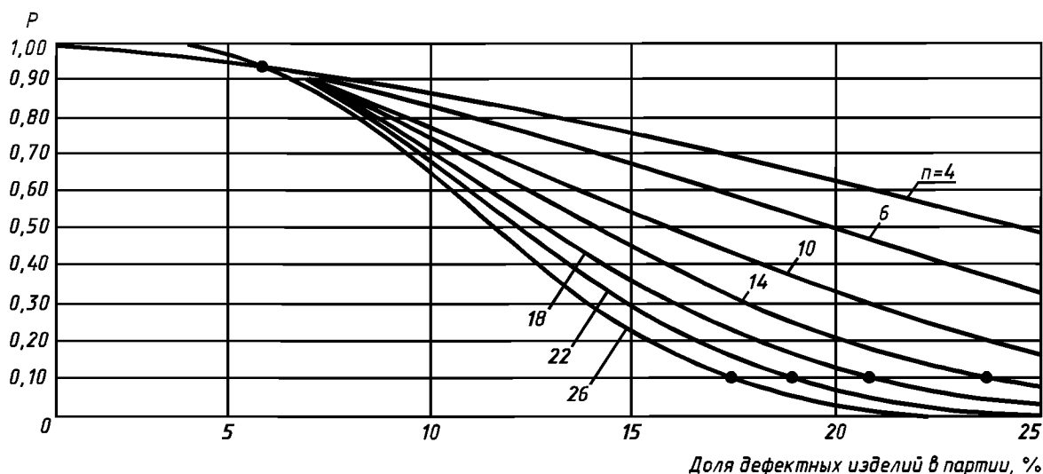
Р и с у н о к 7 — Кривые оперативных характеристик одноступенчатых планов контроля таблицы 9 для AQL = 6,5\% : с установленным односторонним пределом для единичных значений и известным средним квадратическим отклонением 1)
